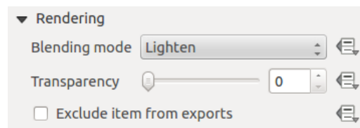
Fig. 14.12: Rendering mode
