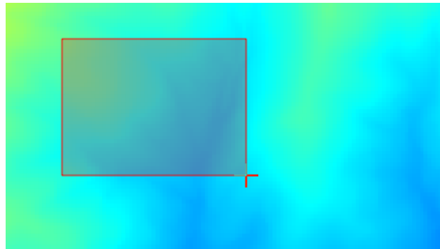
Fig. 19.13: Extent Drag
