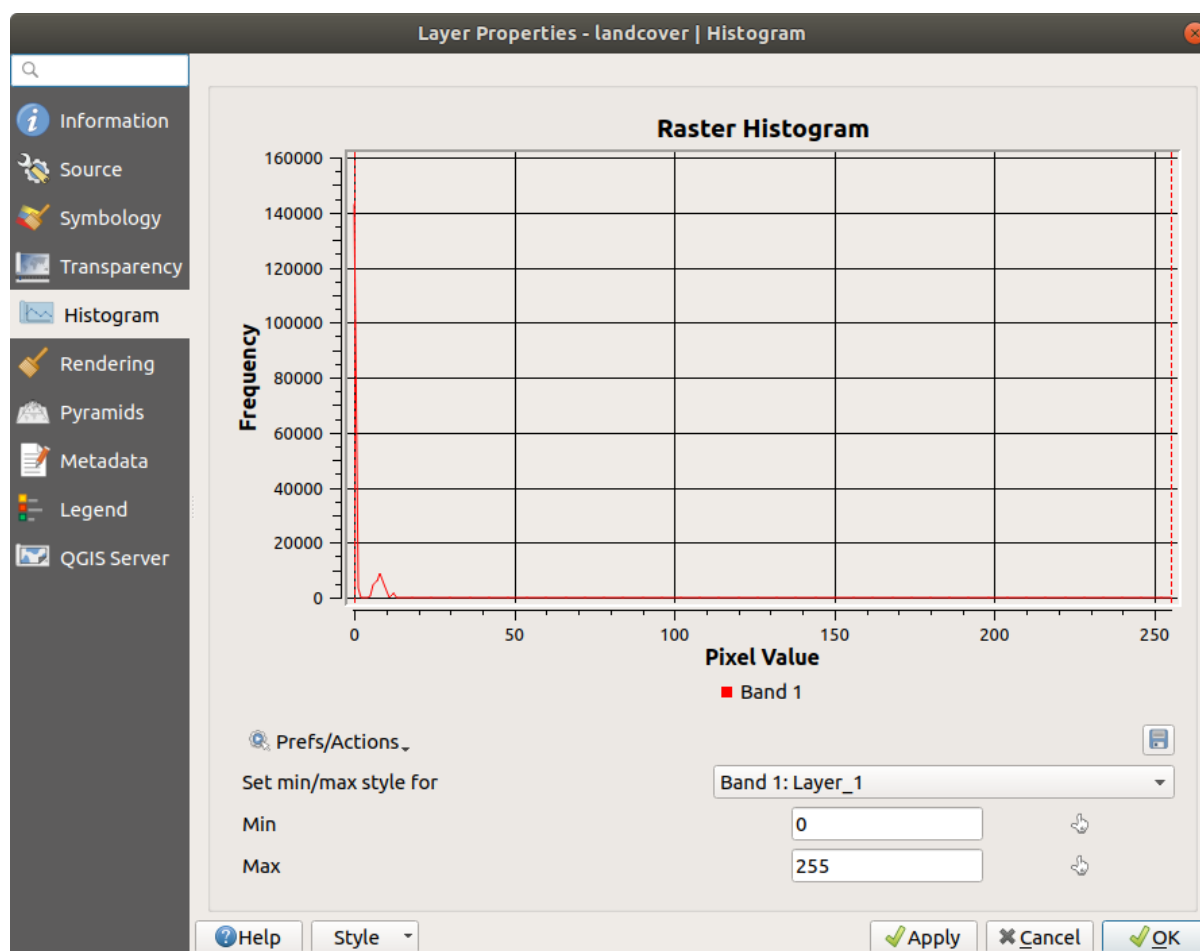
Fig. 13.10: Raster Histogram
