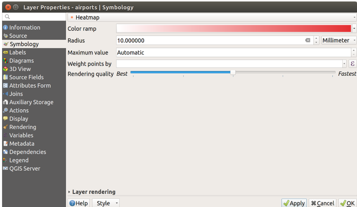
Fig. 12.19: Heatmap dialog
