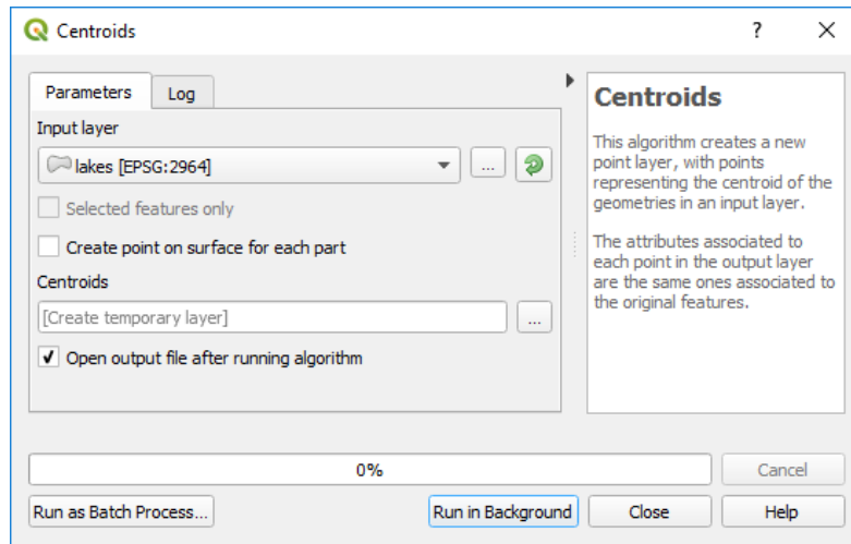
Fig. 19.8: Parameters Dialog
