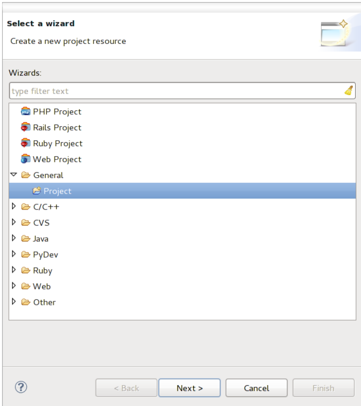
图 16.1: Eclipse project
