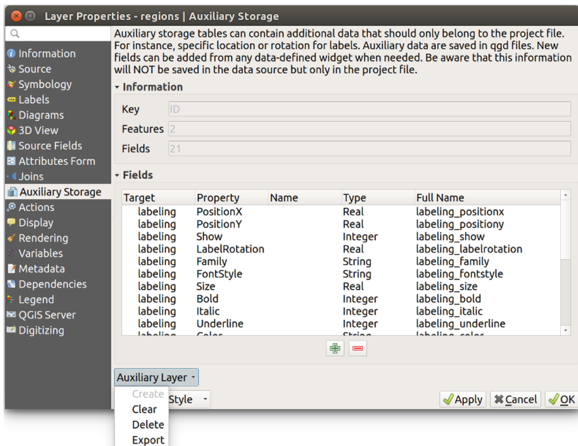
Şekil 14.55: Auxiliary layer management
