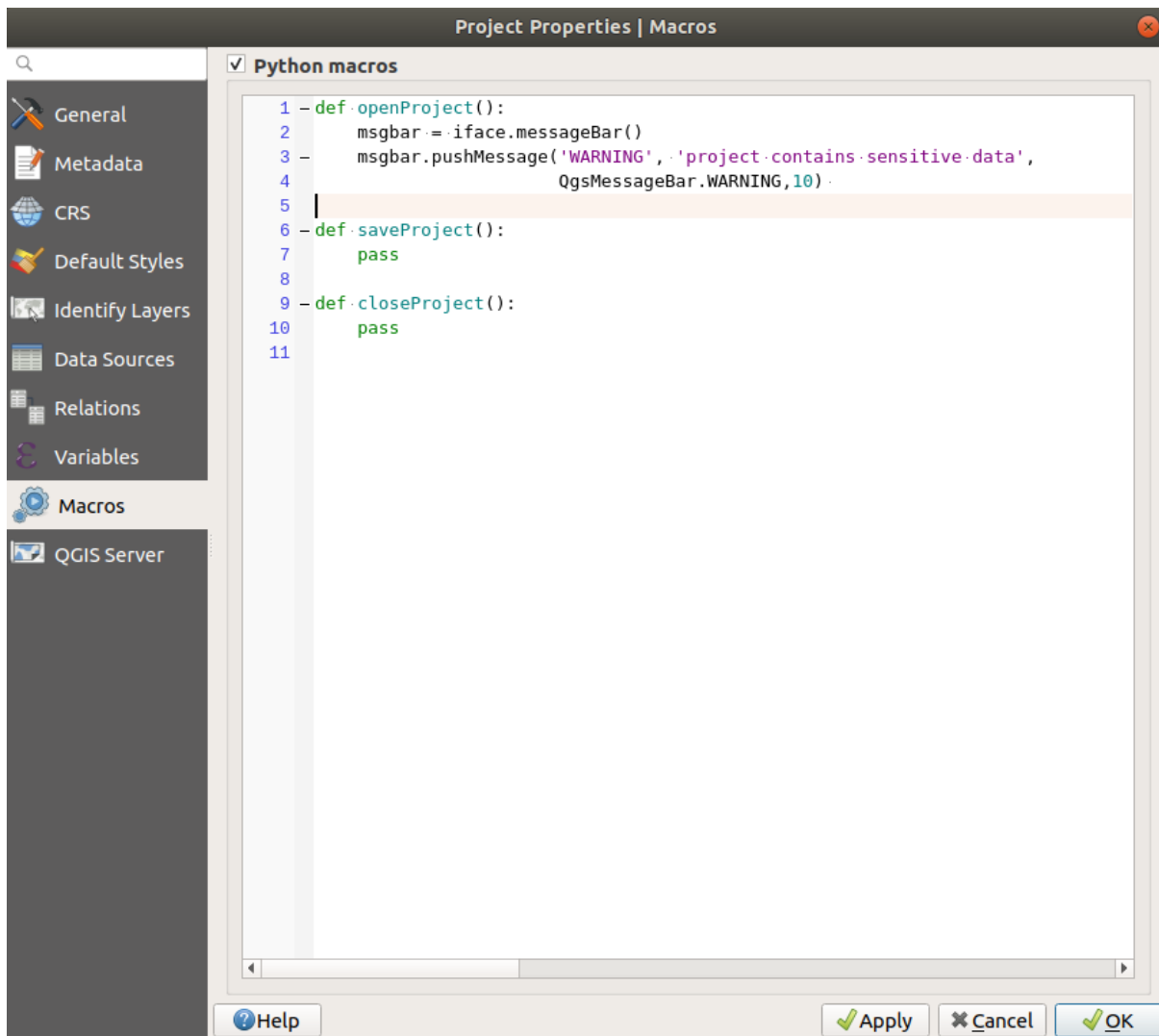
Şekil 9.27: Macro settings in QGIS
