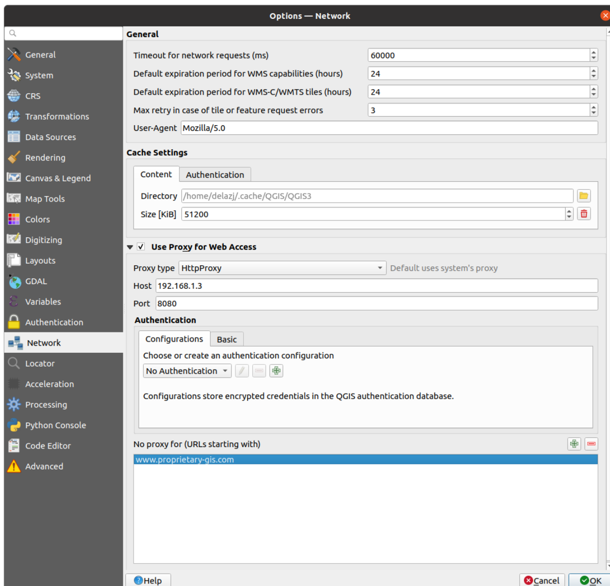
Şekil 9.16: Proxy-settings in QGIS
