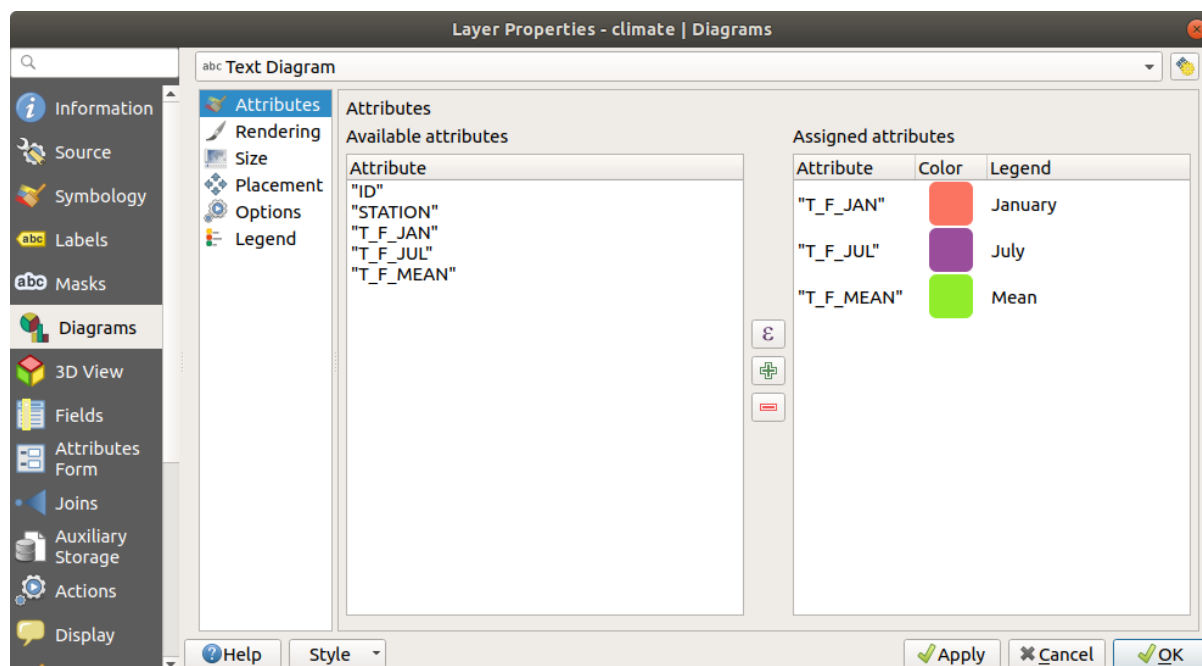
Şekil 14.35: Diagram properties - Attributes tab
