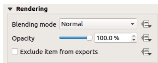
Şekil 18.13: Rendering mode
