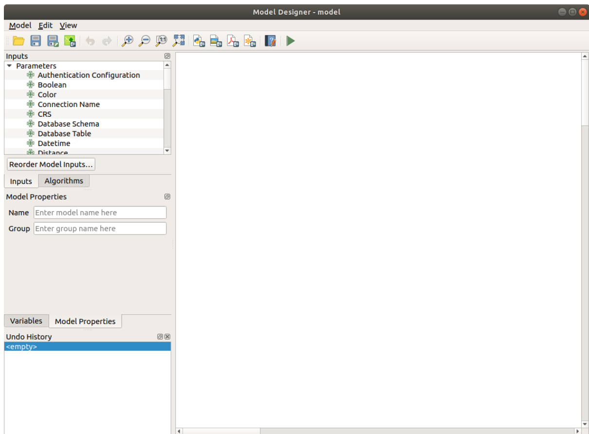
Şekil 23.16: Modeler
