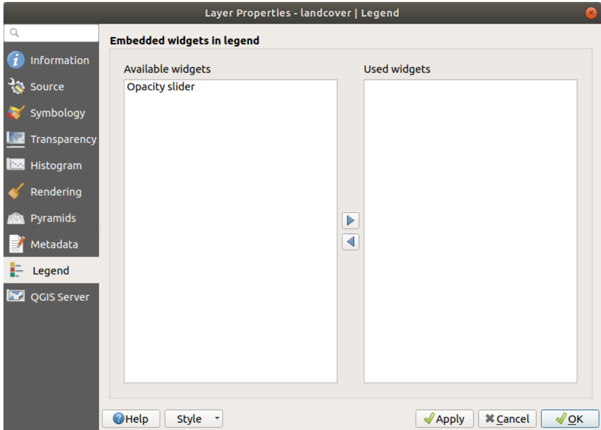
Şekil 15.15: Raster Legend
