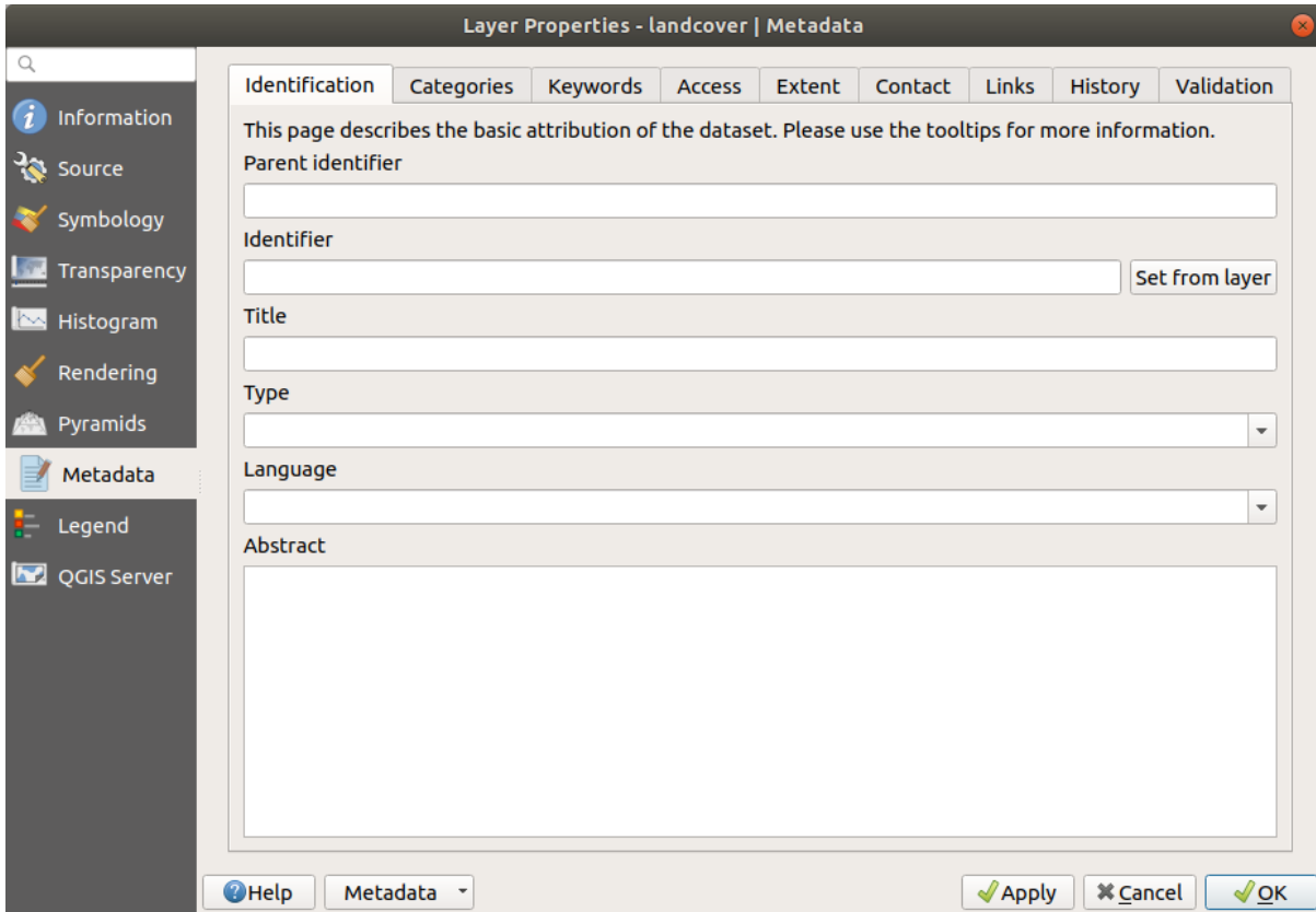
Şekil 15.14: Raster Metadata
