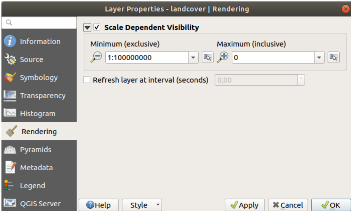
Şekil 15.12: Raster Rendering
