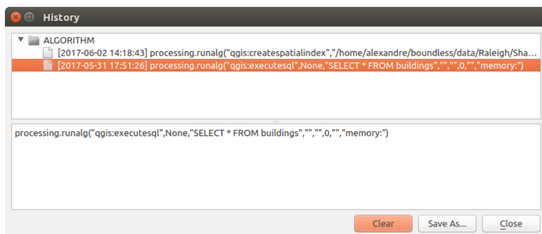
Şekil 23.15: History
