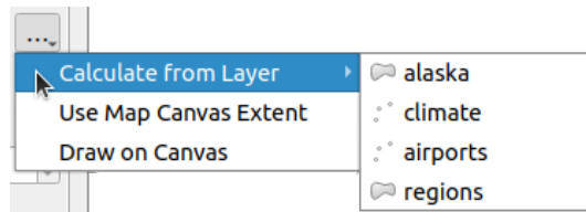
Şekil 23.11: Extent selector
