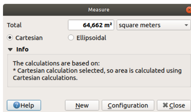
Şekil 11.18: Measure Area
