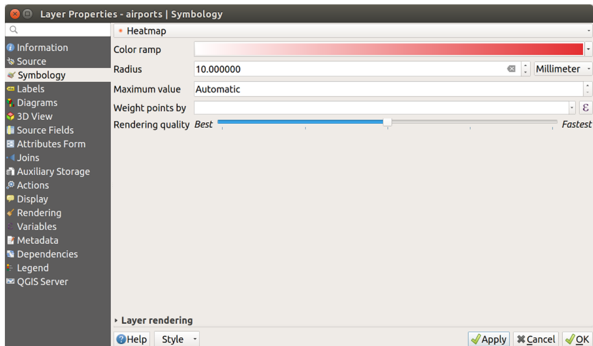
Şekil 14.12: Heatmap dialog
