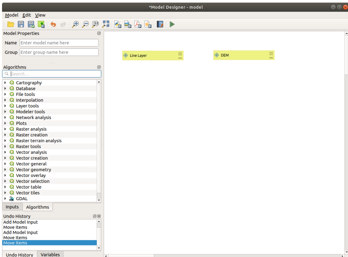
Şekil 23.19: Model Inputs
