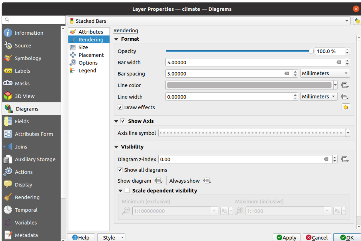
Şekil 14.36: Diagram properties - Rendering tab
