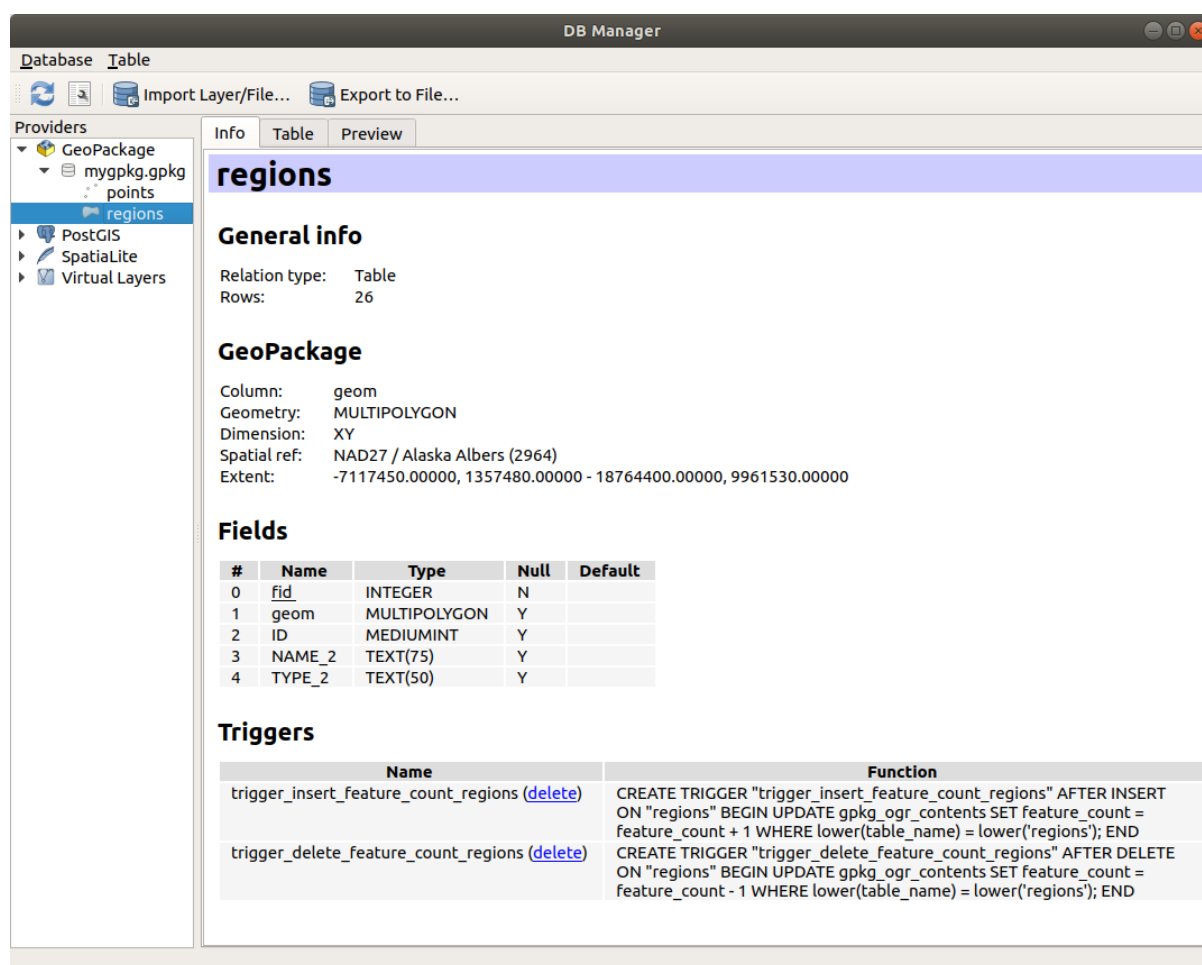
Şekil 13.3: DB Manager dialog
