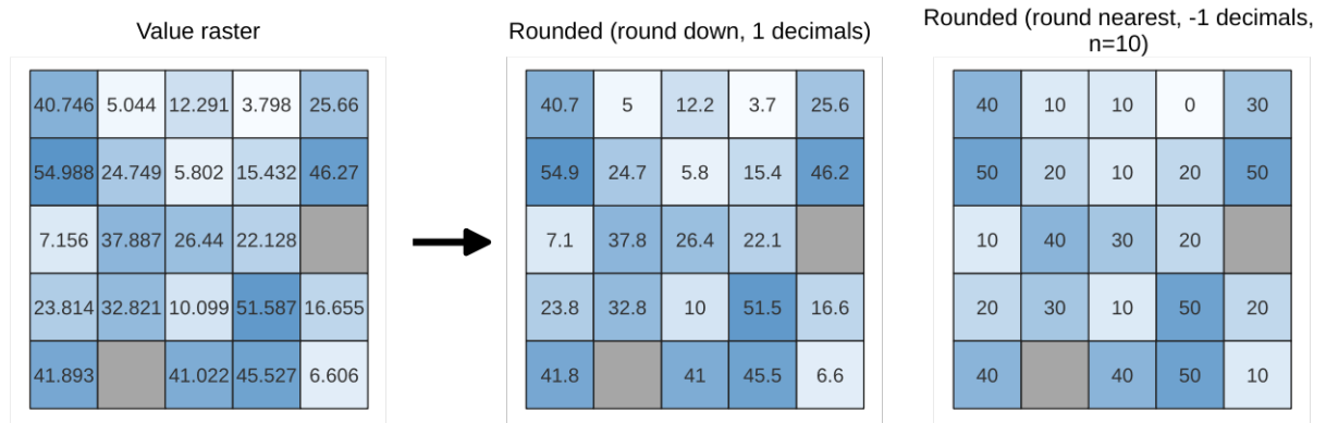
Şekil 24.14: Rounding values of a raster
