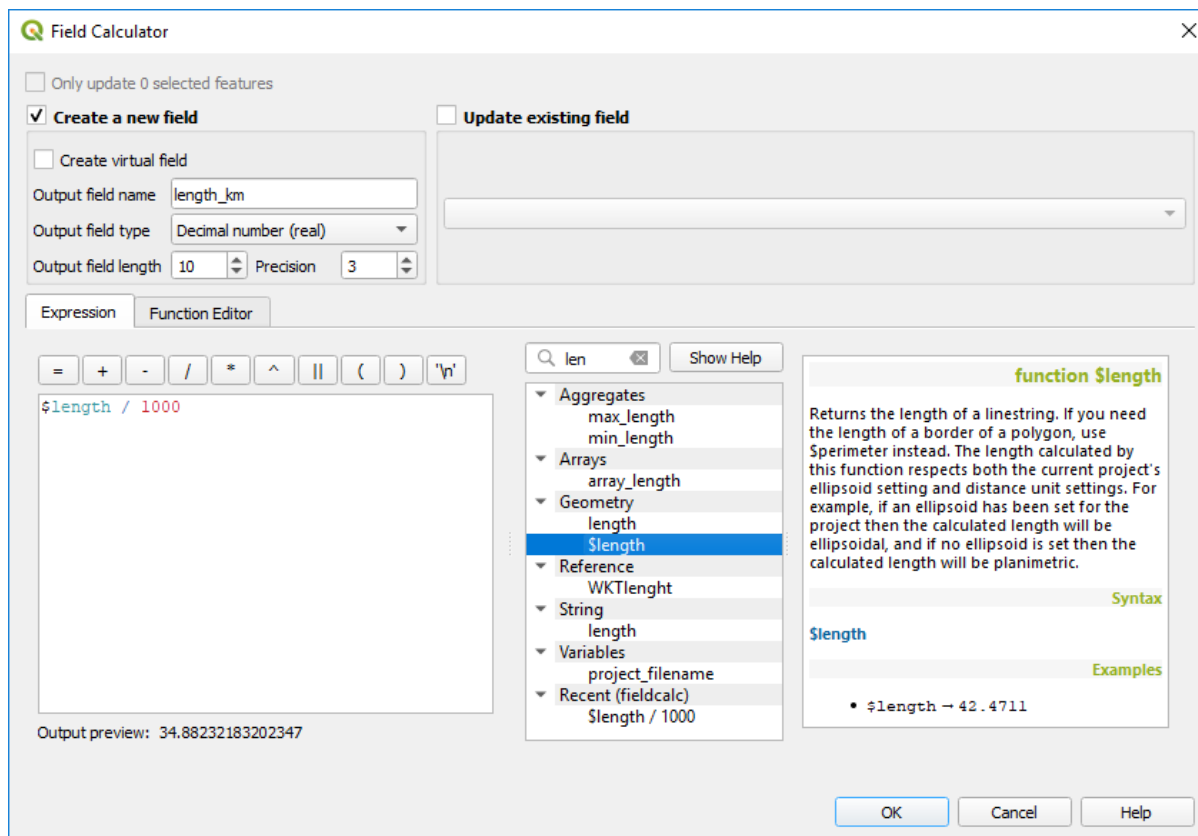
Şekil 14.73: Field Calculator
