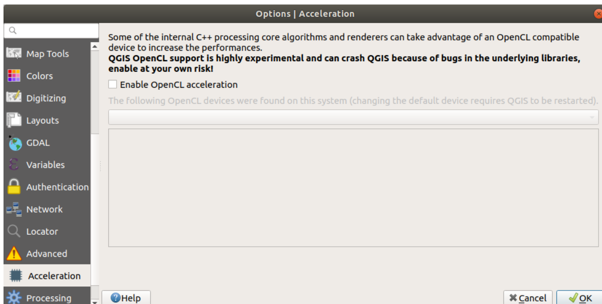
Şekil 9.19: Acceleration tab
