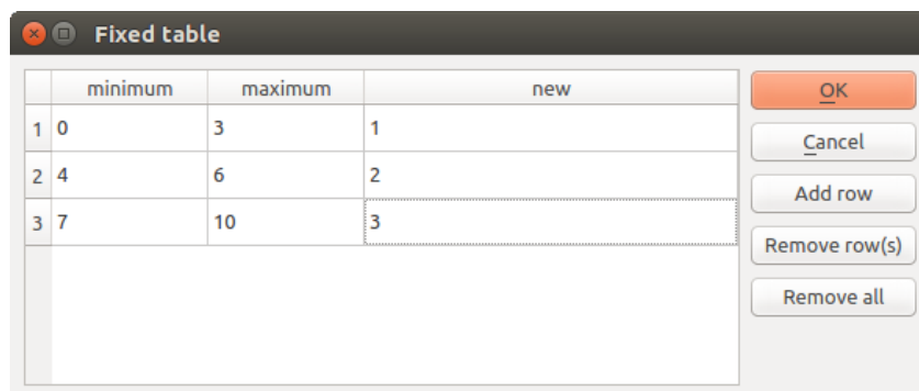
Şekil 23.13: Fixed Table
