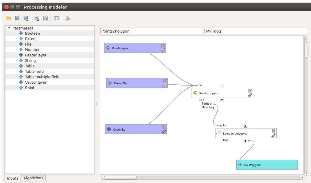
Şekil 23.2: Processing Modeler
