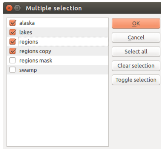
Şekil 23.12: Multiple Selection
