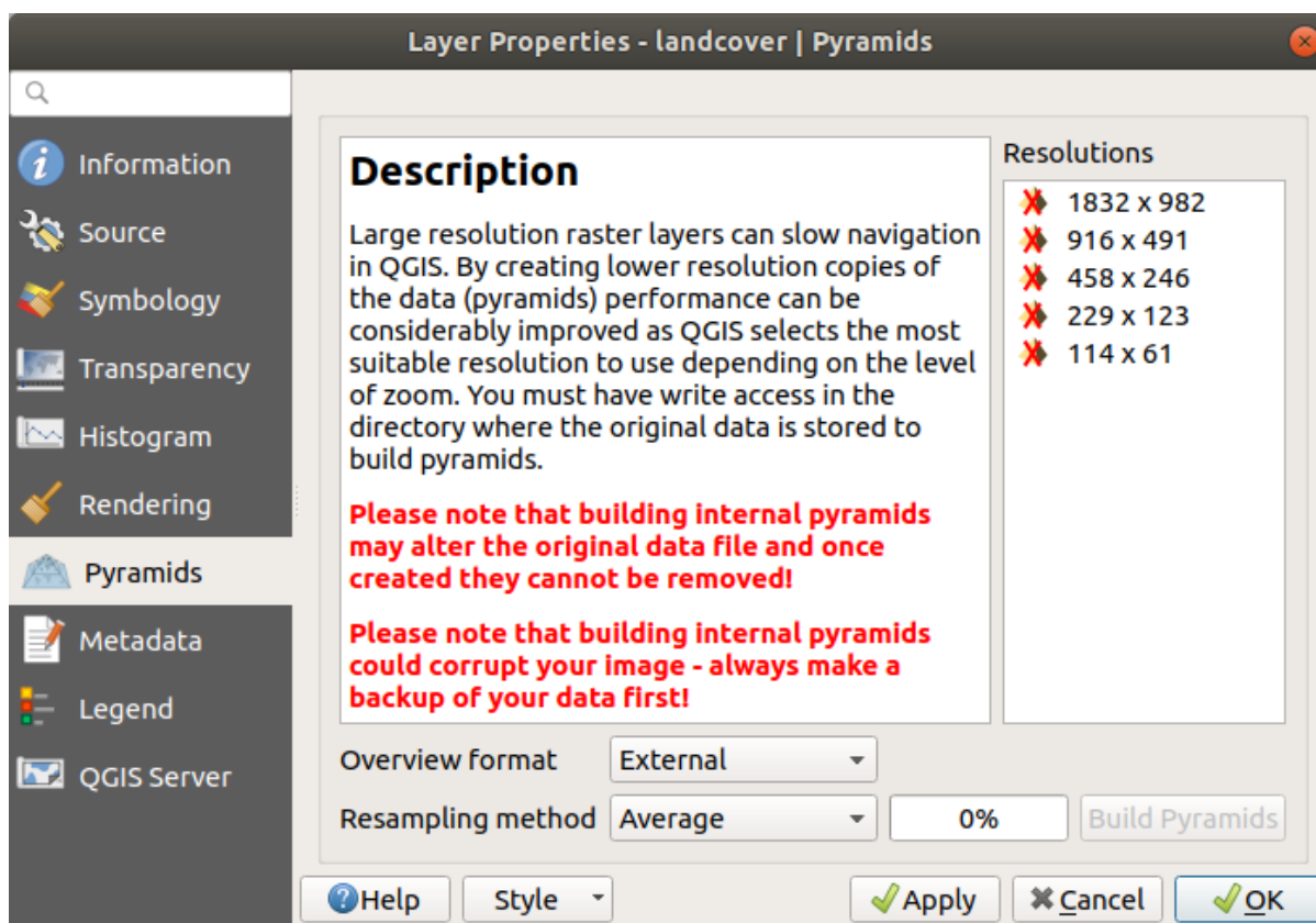
Şekil 15.13: Raster Pyramids
