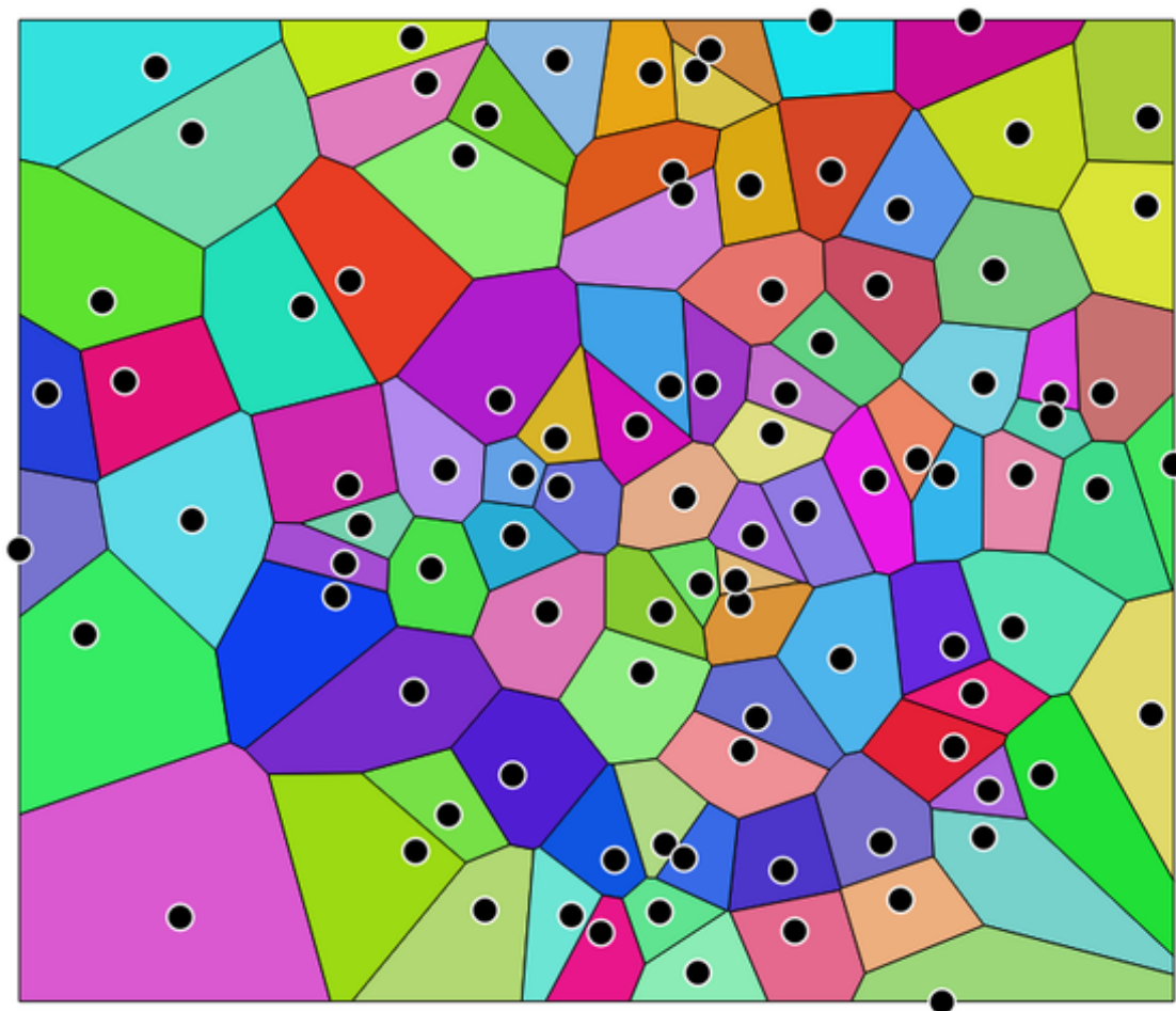
Şekil 24.91: Voronoi polygons
