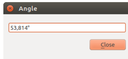
Şekil 11.19: Measure Angle
