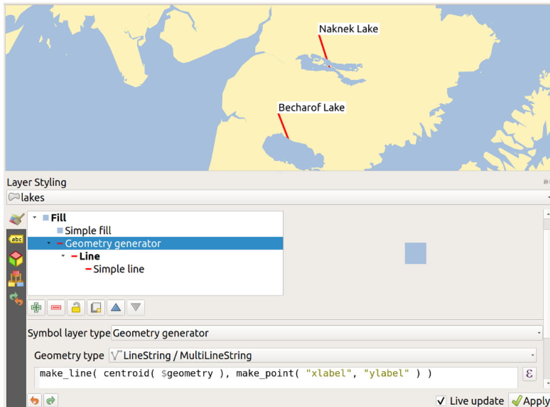
Şekil 14.34: Moved labels
