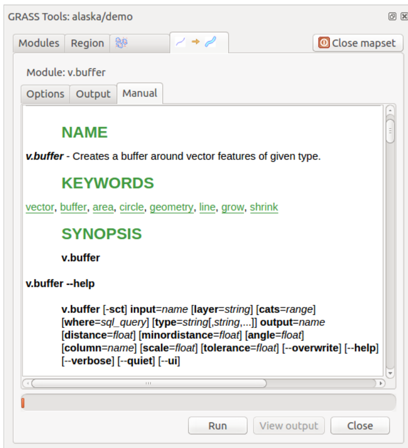
Şekil 22.6: GRASS Toolbox Module Manual
