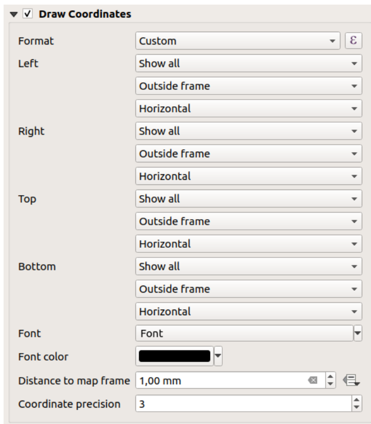
Şekil 18.20: Grid Draw Coordinates dialog
