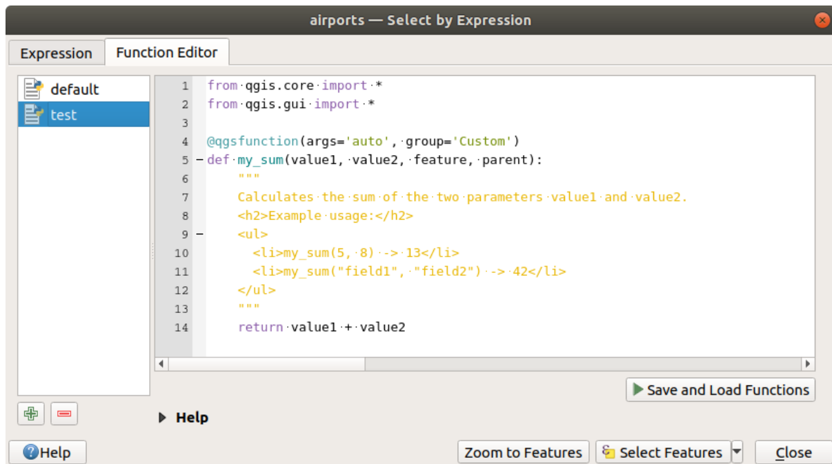
Рис. 14.66: The Function Editor tab
