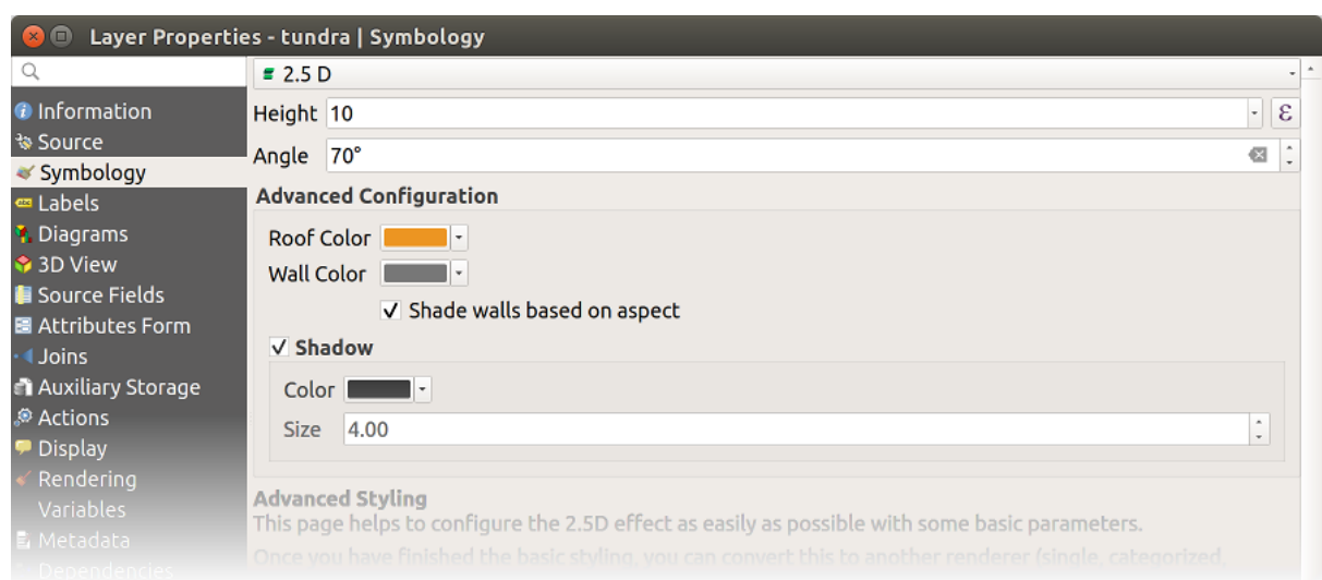
Рис. 14.13: 2.5D dialog
