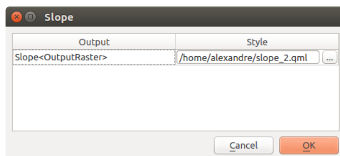
Рис. 23.5: Rendering Styles
