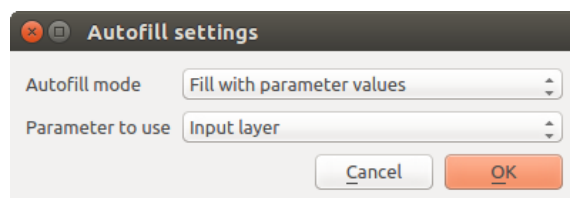
Рис. 23.32: Диалог автозаполнения
