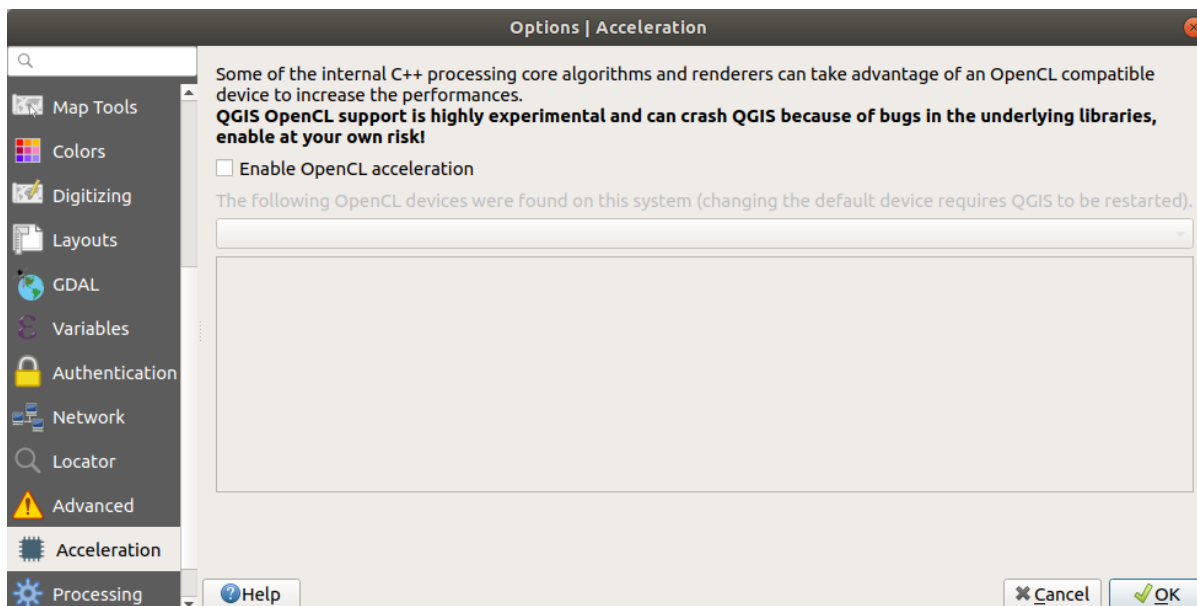
Рис. 9.19: Acceleration tab
