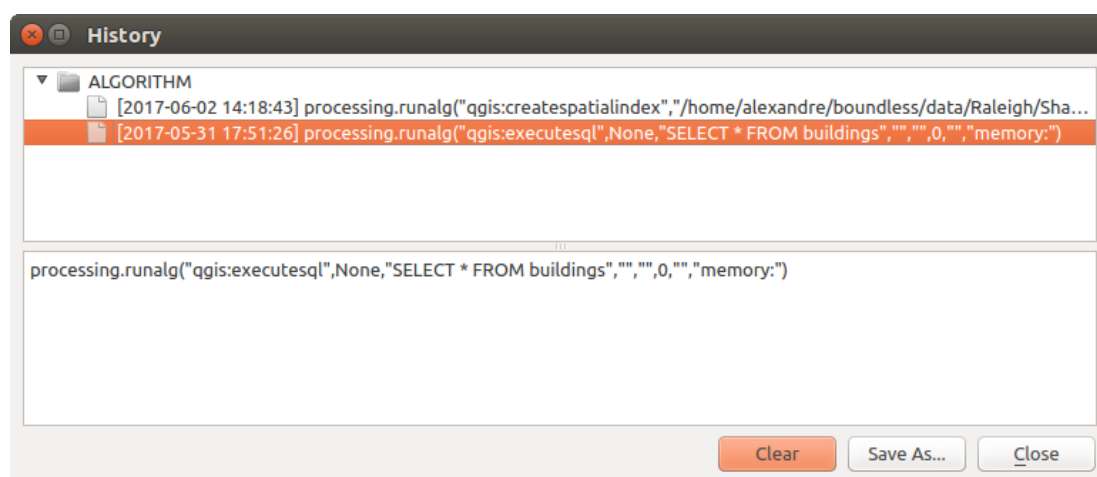
Рис. 23.15: History
