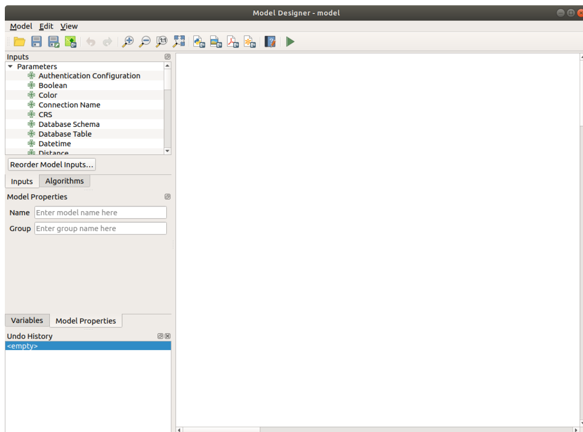
Рис. 23.16: Modeler
