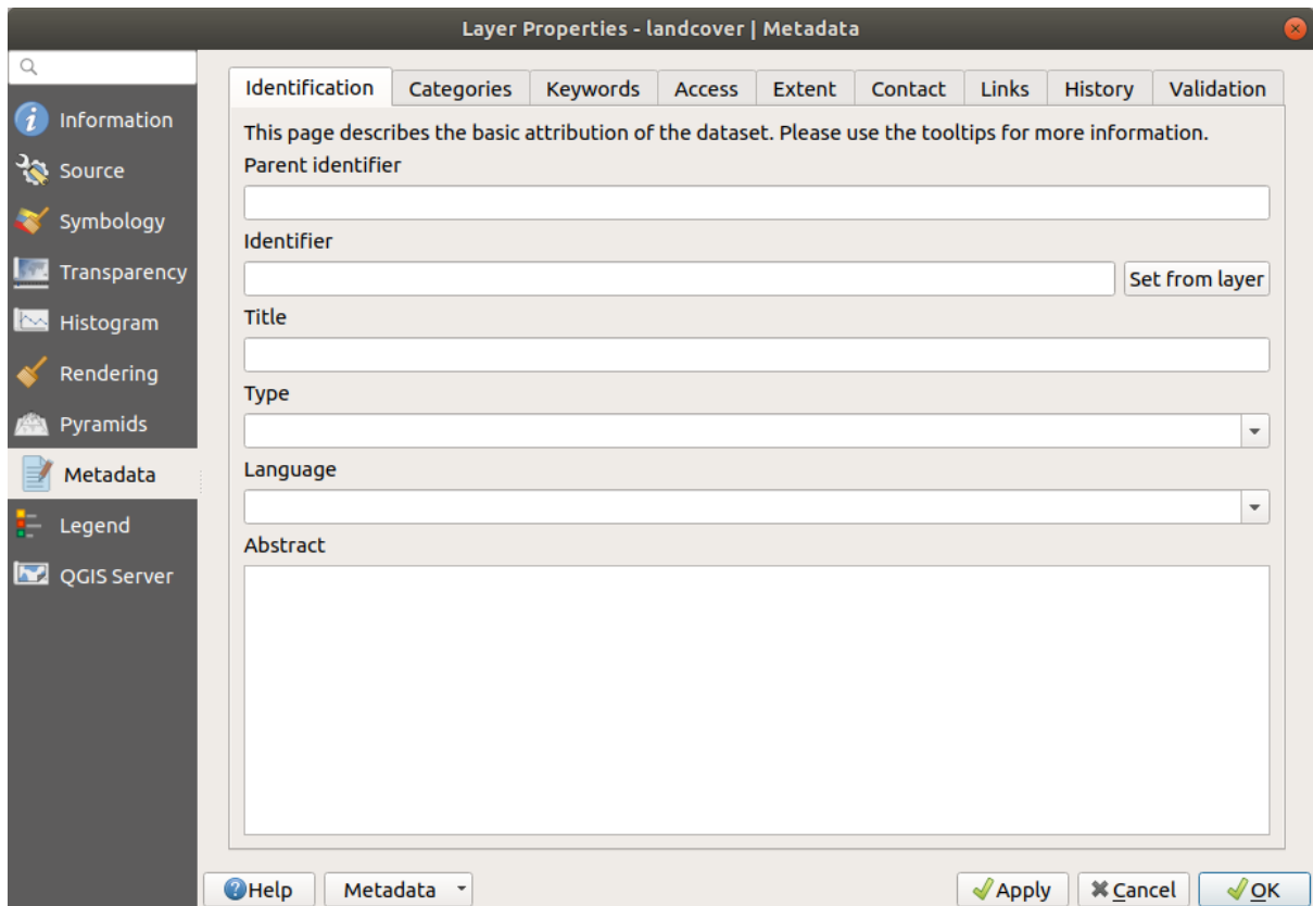
Рис. 15.14: Raster Metadata
