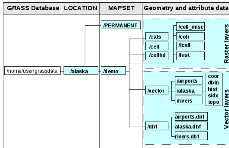
Рис. 22.1: Данные GRASS в районе «alaska»
