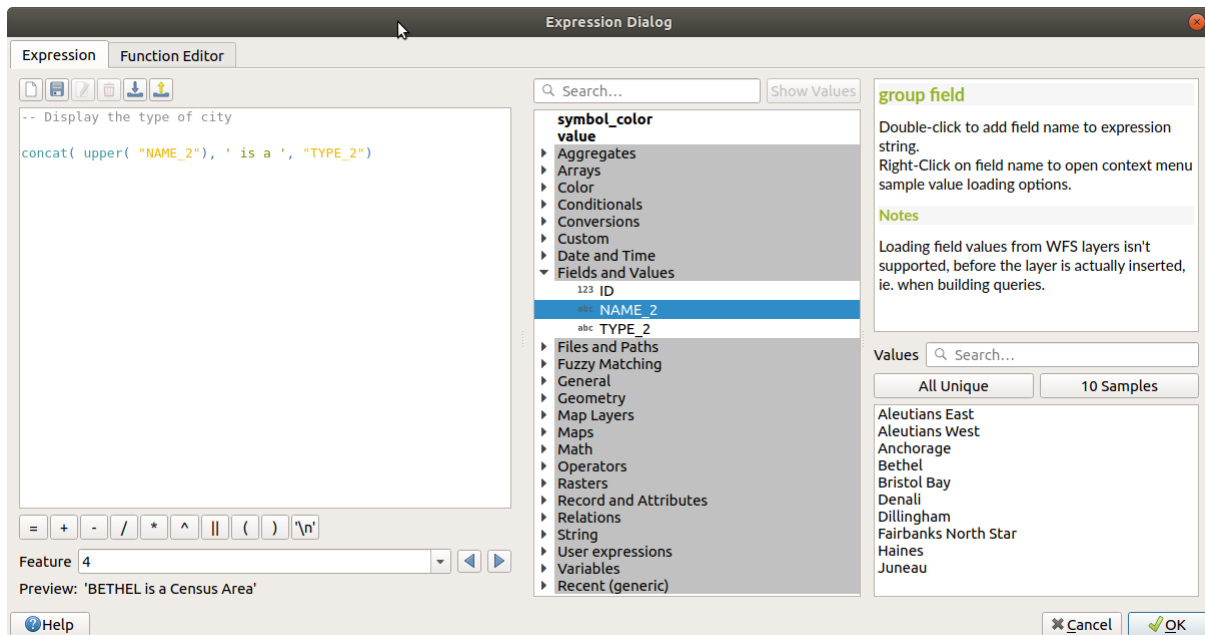
Рис. 14.65: The Expression tab
