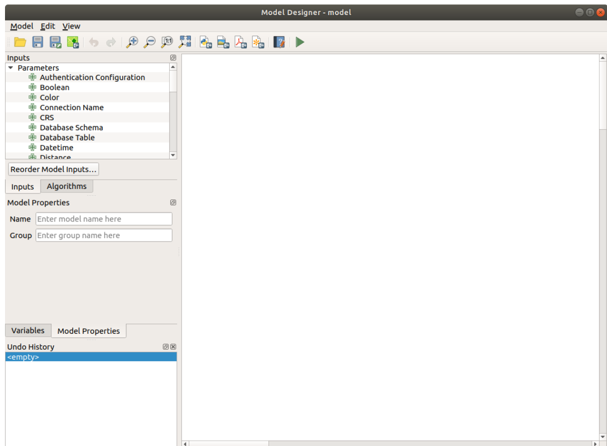
Fig. 23.16: Modeler
