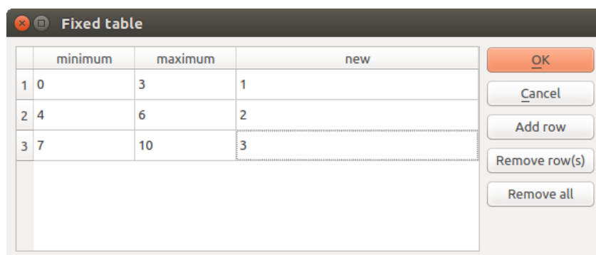
Fig. 23.13: Fixed Table
