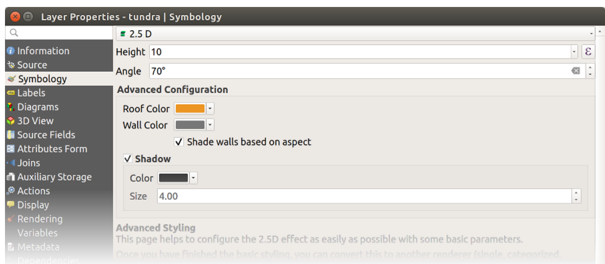
Fig. 14.13: 2.5D dialog
