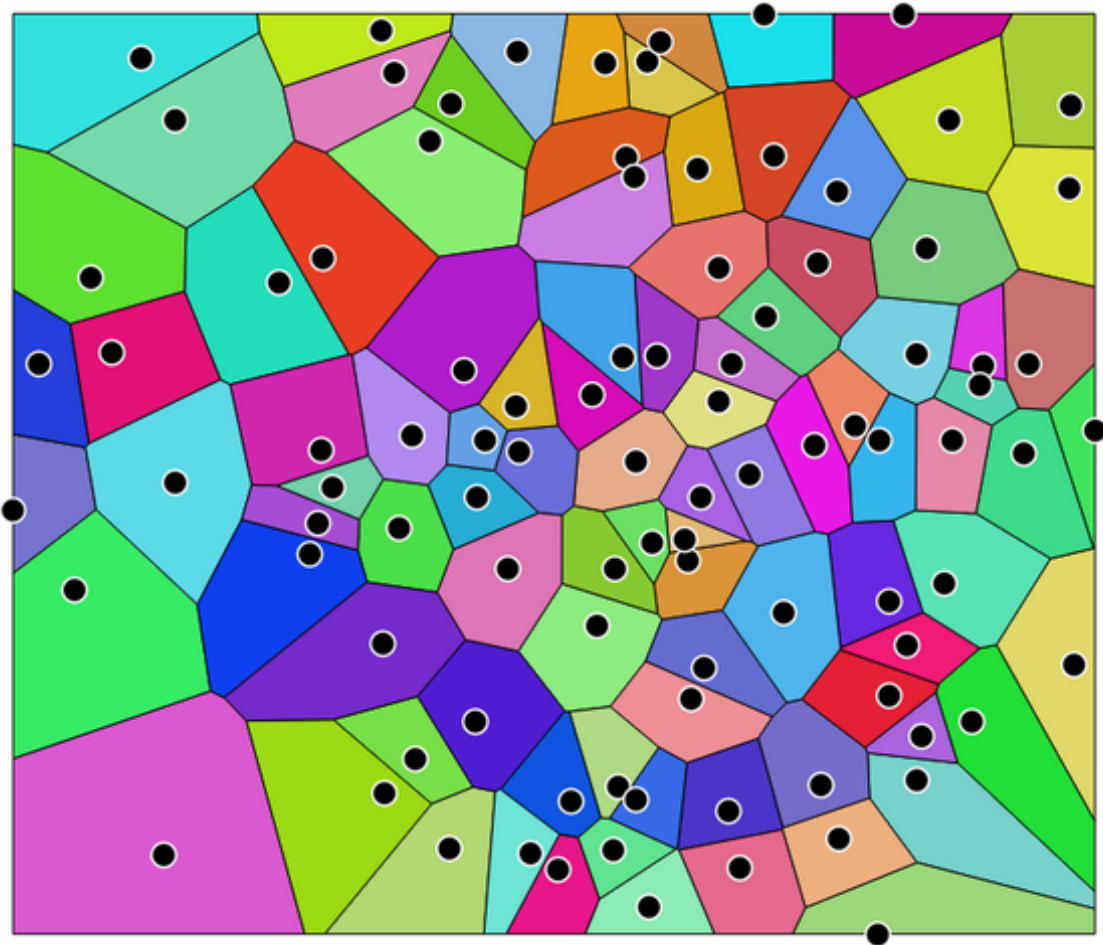
图 23.77: Voronoi polygons
