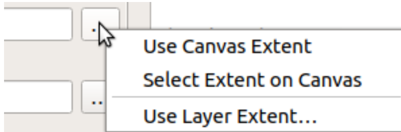
图 22.11: Extent selector
