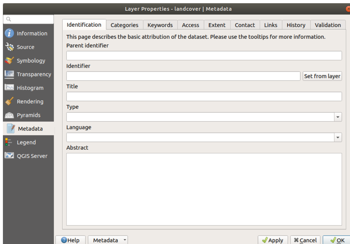
图 15.13: Raster Metadata
