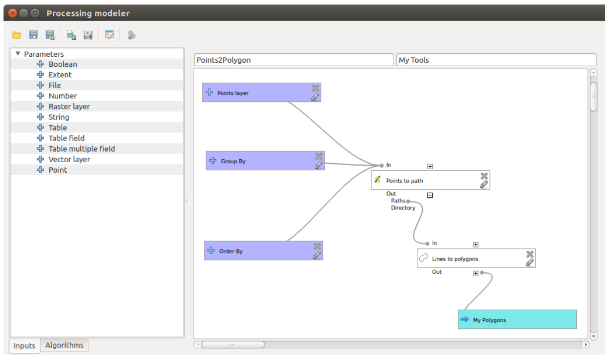
图 22.2: 处理模型
