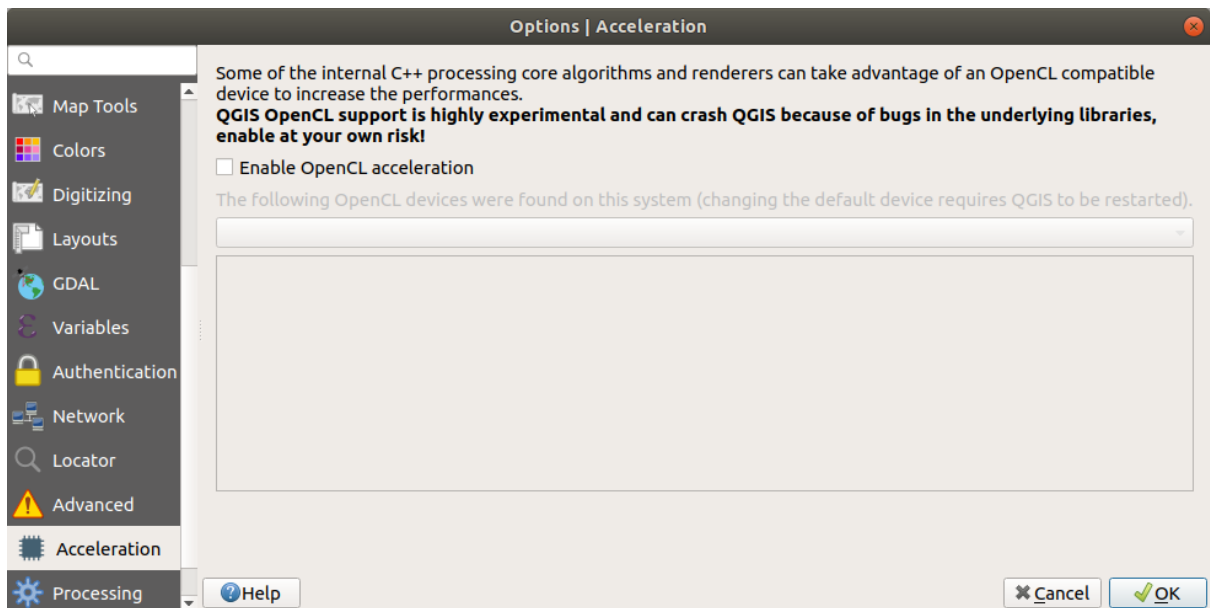
图 9.18: Acceleration tab
