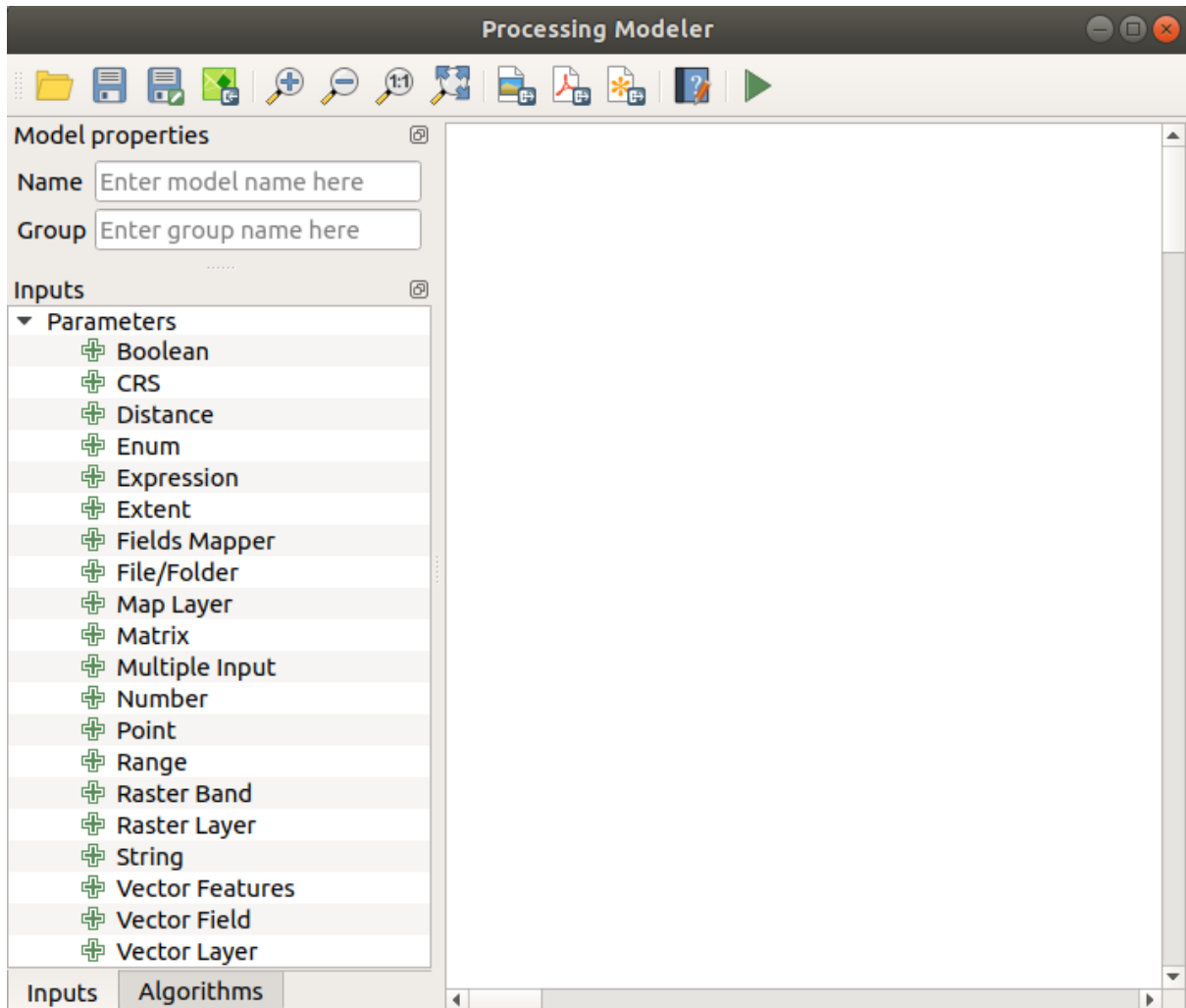
图 22.18: Modeler
