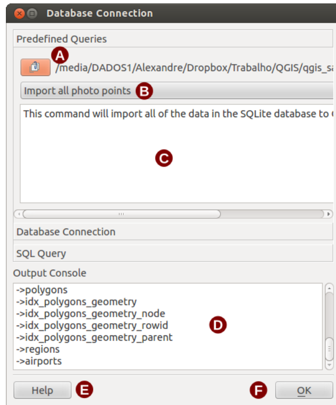
Şekil 24.16: The eVis Predefined Queries tab
