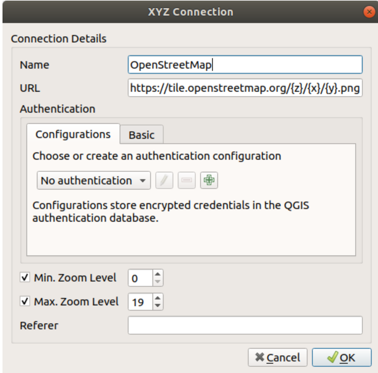
Şekil 13.12: XYZ Tiles - OpenStreetMap configuration
