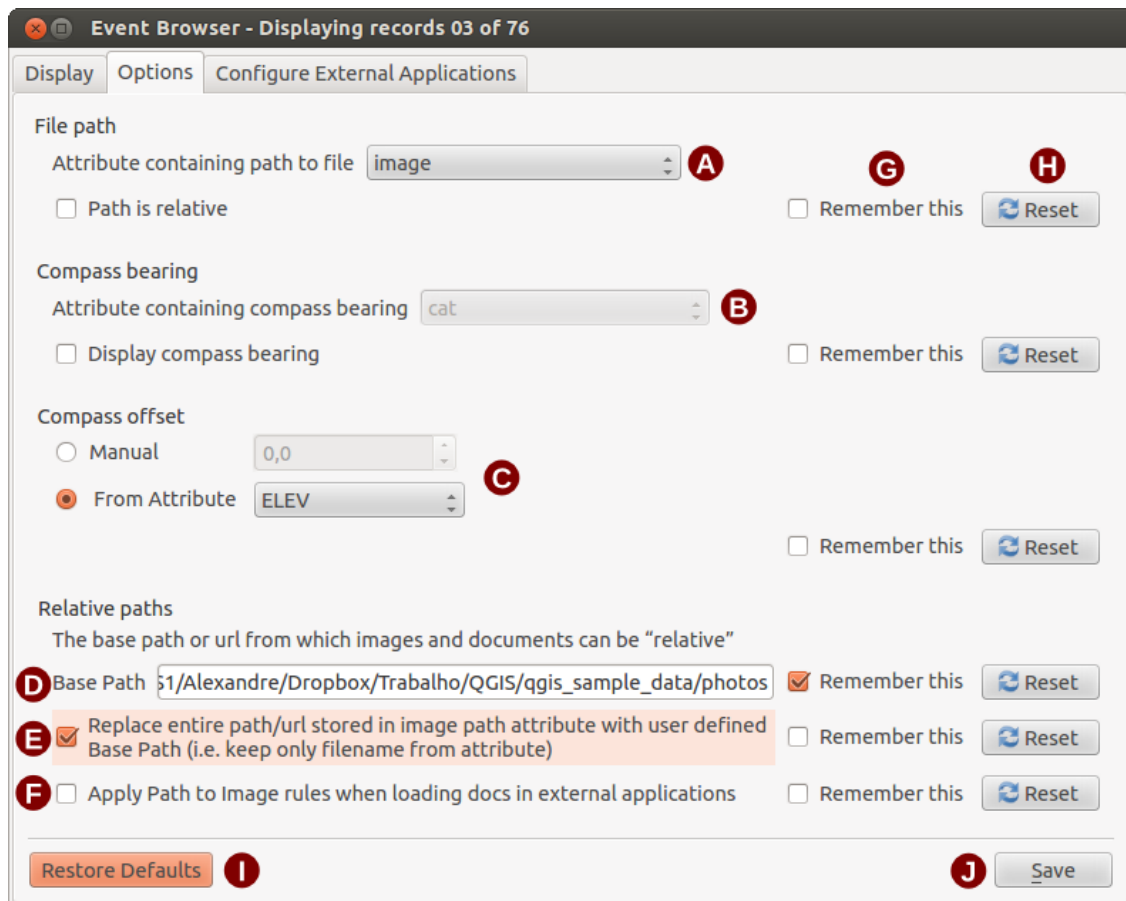
Şekil 24.12: The eVis Options window
