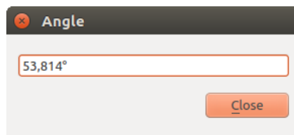
Şekil 11.19: Measure Angle
