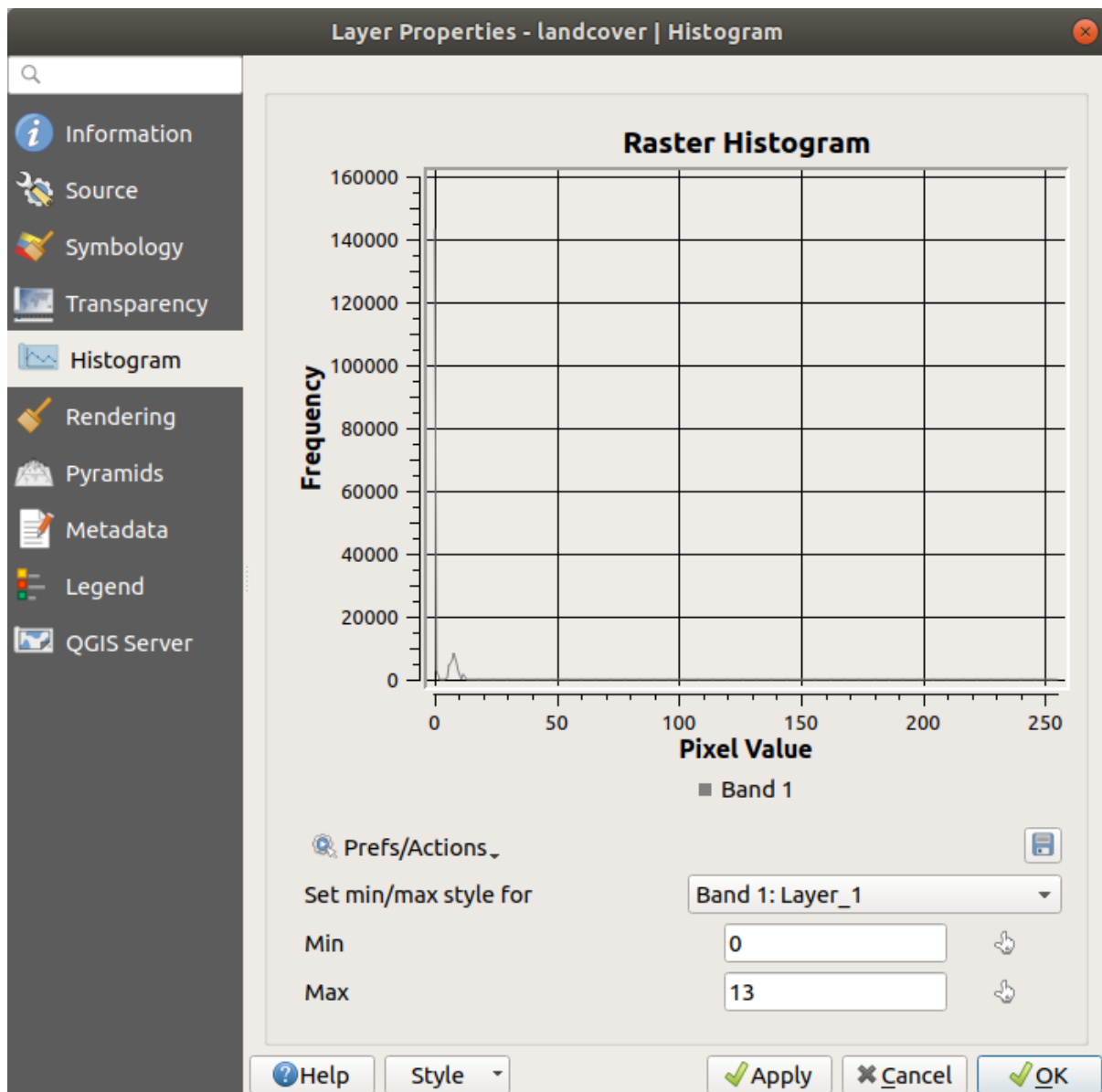
Şekil 15.10: Raster Histogram
