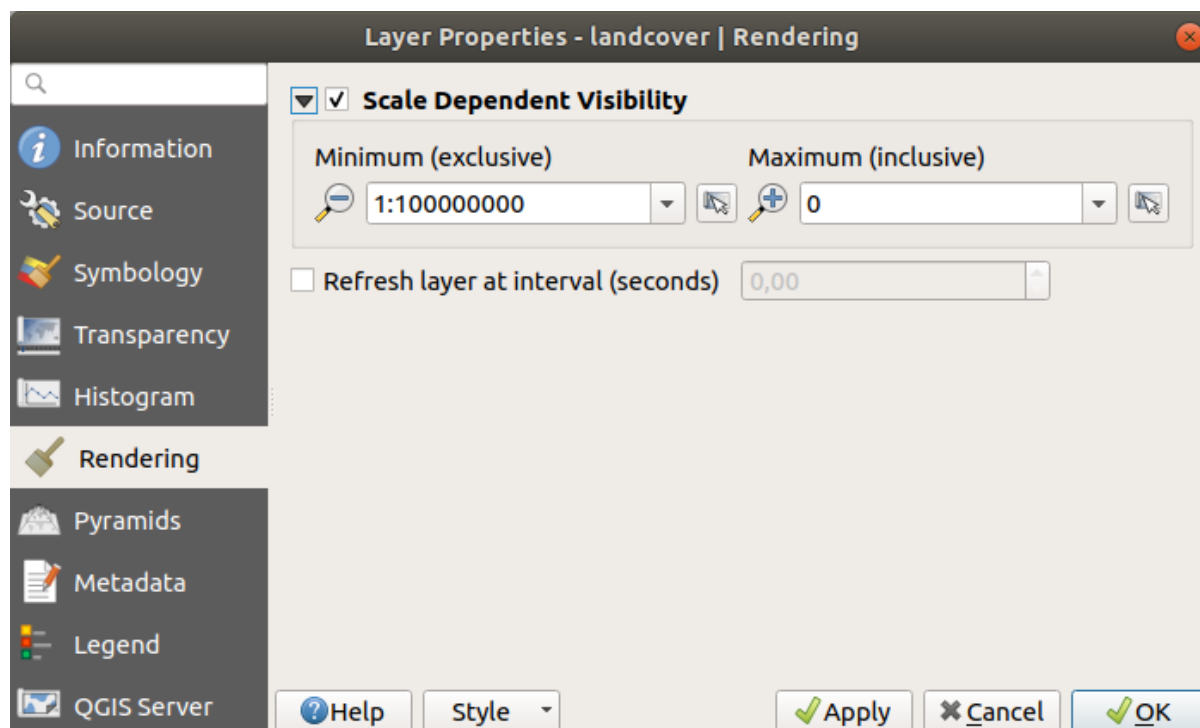
Şekil 15.11: Raster Rendering
