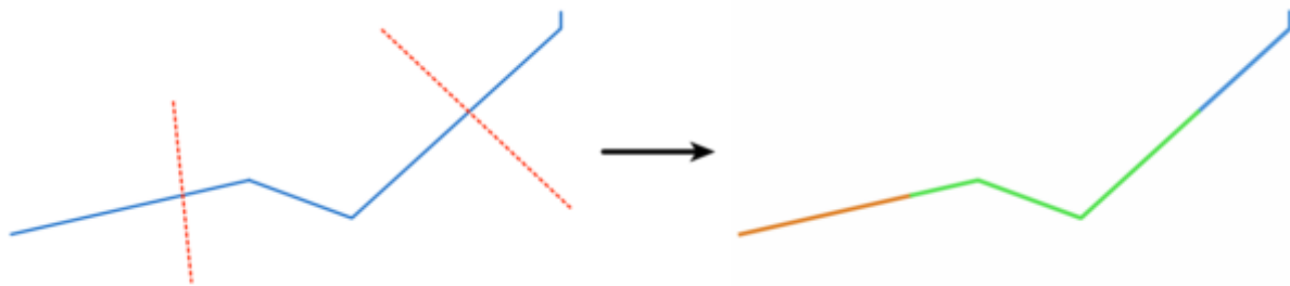
Şekil 23.82: Split lines
