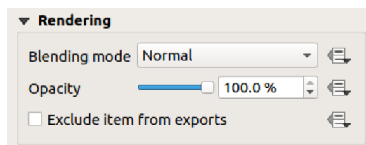
Şekil 17.13: Rendering mode
