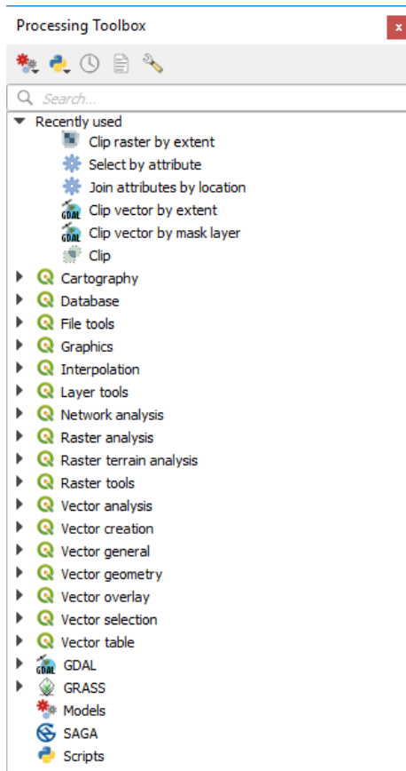
Şekil 22.1: Processing Toolbox
