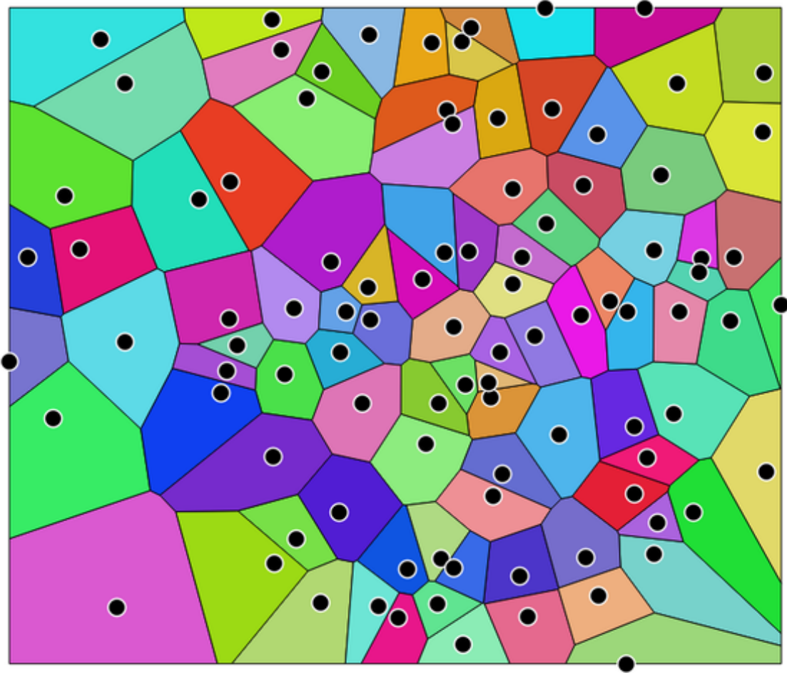
Şekil 23.77: Voronoi polygons
