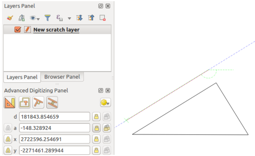
Şekil 14.100: Parallel digitizing
