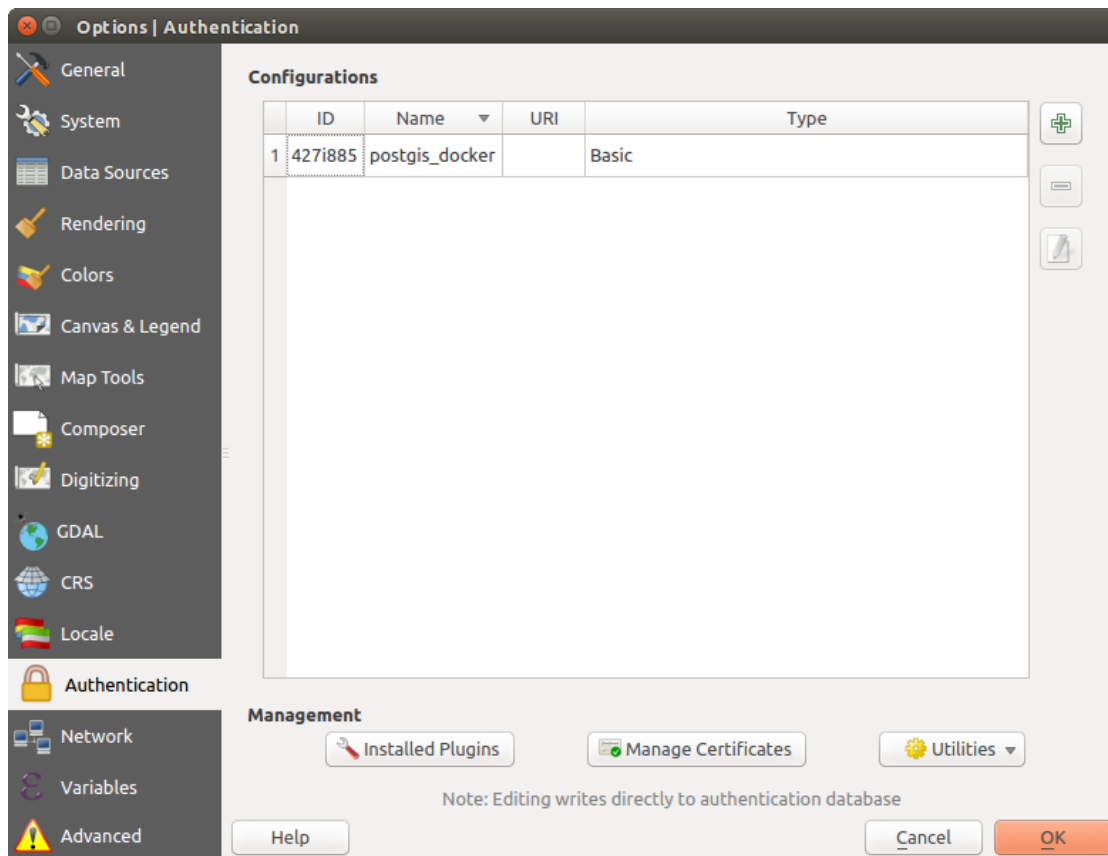
Şekil 20.5: Configurations editor
