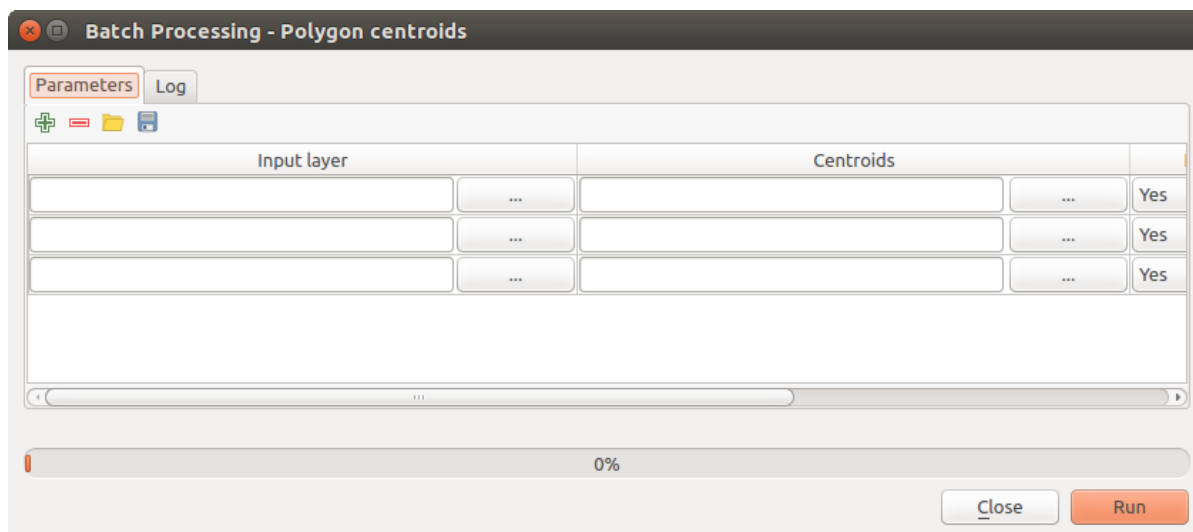
Şekil 22.30: Batch Processing
