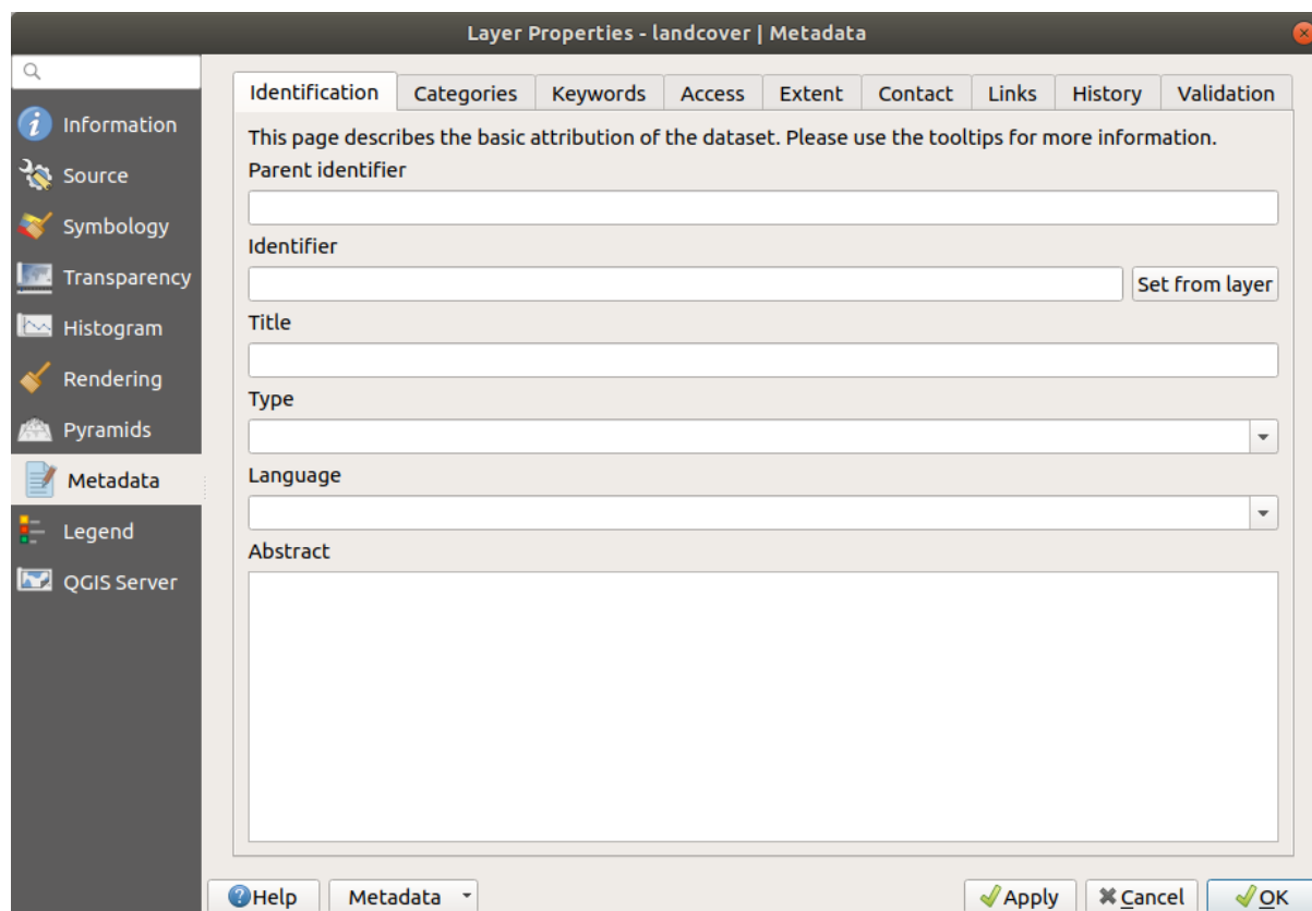
Şekil 15.13: Raster Metadata
