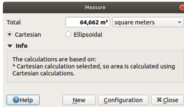
Şekil 11.18: Measure Area
