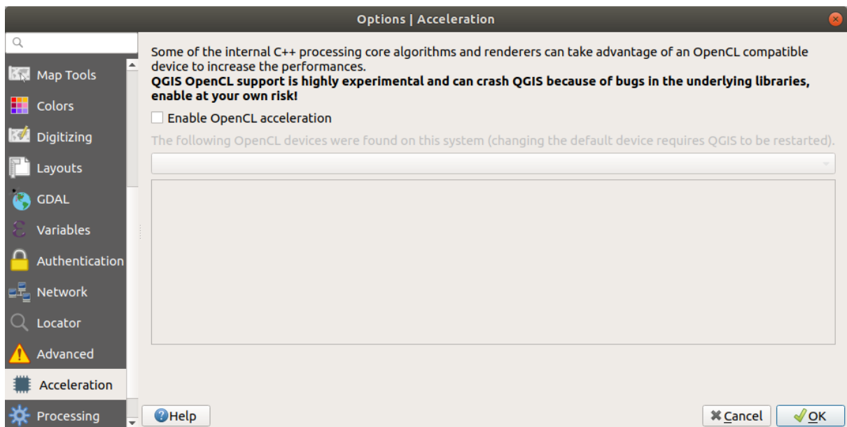
Şekil 9.18: Acceleration tab
