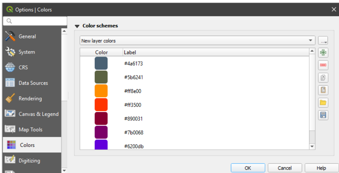
Şekil 9.7: Colors Settings
