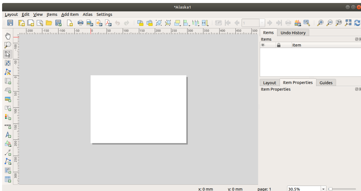
Şekil 17.2: Print Layout
