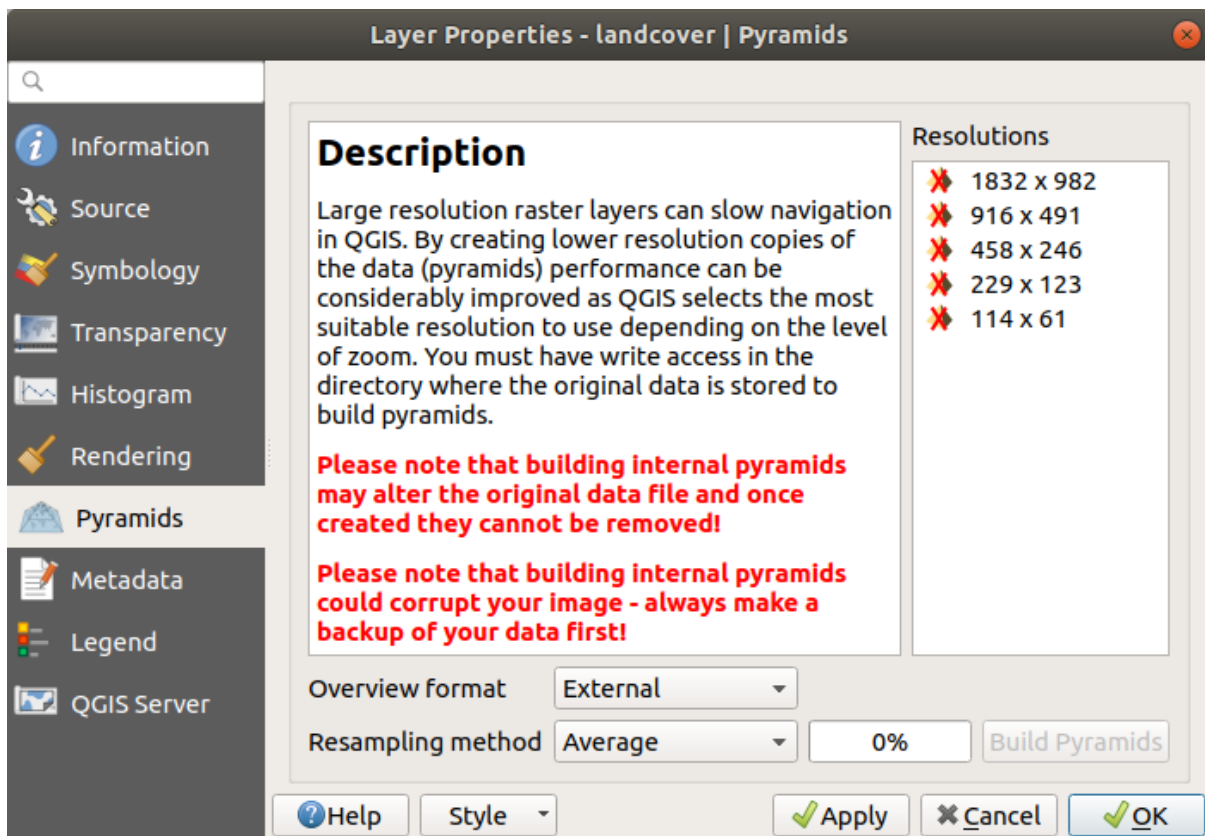
Şekil 15.12: Raster Pyramids
