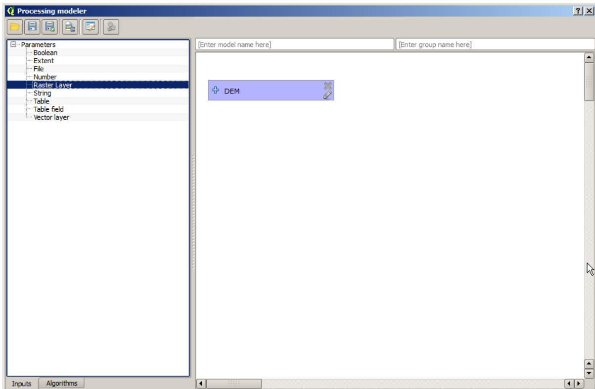
Kuva 17.19: Model Parameters
