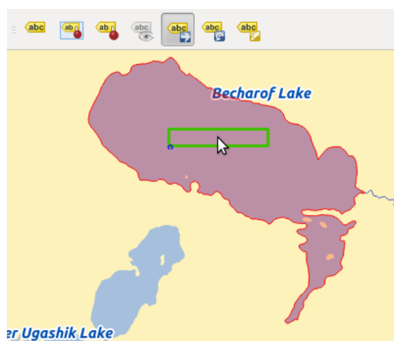
Kuva 12.20: Move labels 🐧
