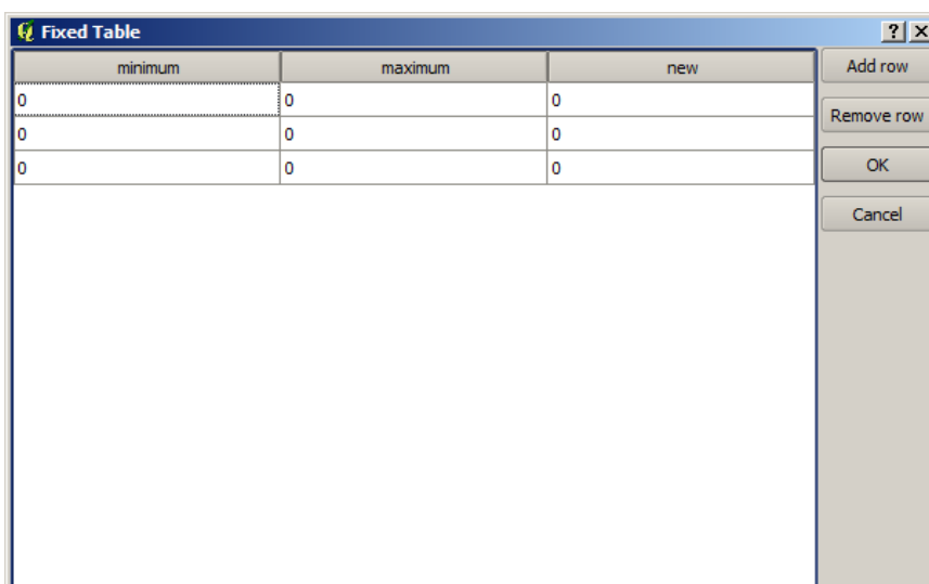
Kuva 17.14: Fixed Table
