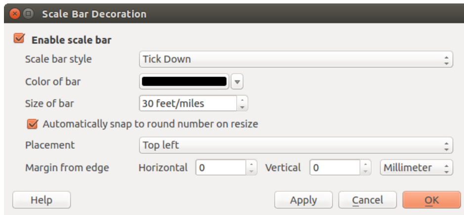
Figure 8.21: Dialog měřítka
