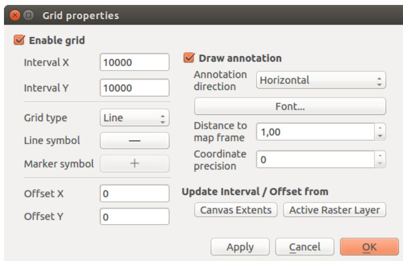
Figure 8.18: Dialog mřížky
