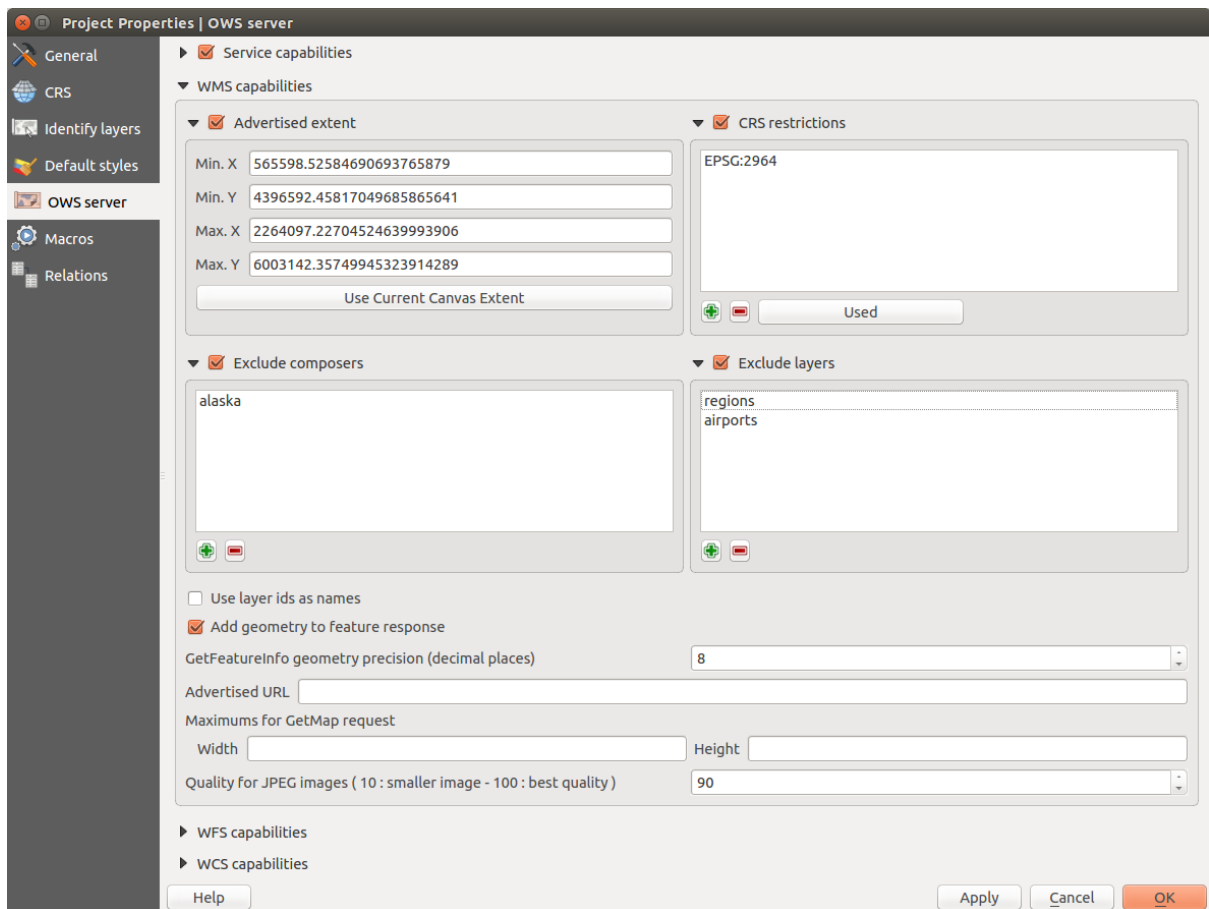
Figure 14.5: Määrietykset QGIS Palvelimen WMS/WFS/WCS projektille
