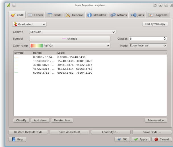
Kuva 11.10: Graduated Symbolizing options 🐧
