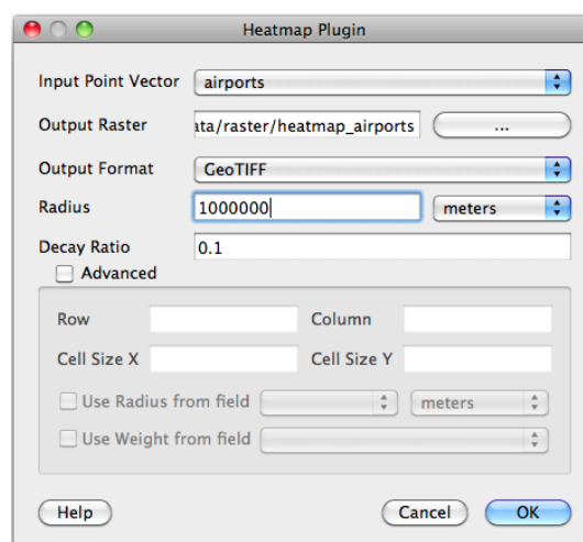
Kuva 19.29: The Heatmap Dialog X
