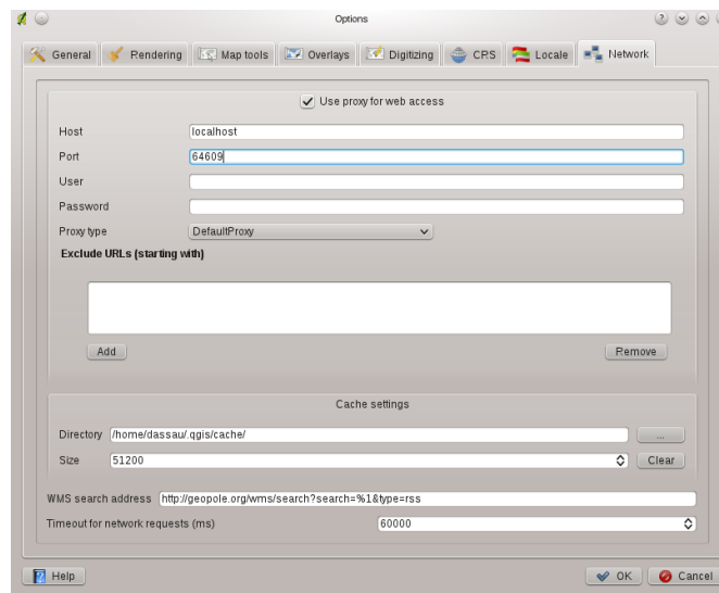
Kuva 8.2: Proxy-settings in QGIS
