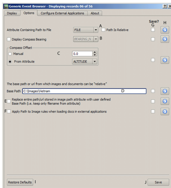
Kuva 19.10: The eVis Options window
